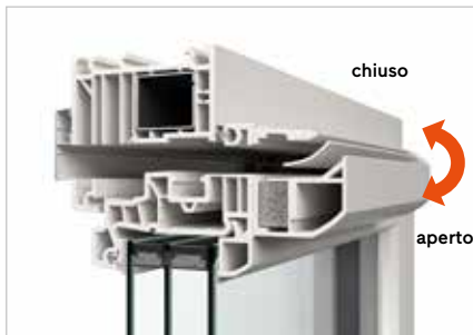
PassiveVent Midi: applicato sull'anta con controllo dell'umidità
