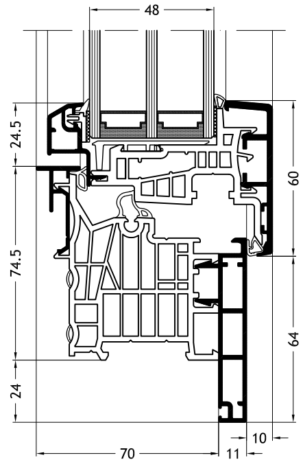
Blendrahmen L-Form D1X mit Flügel Classic-line A27
