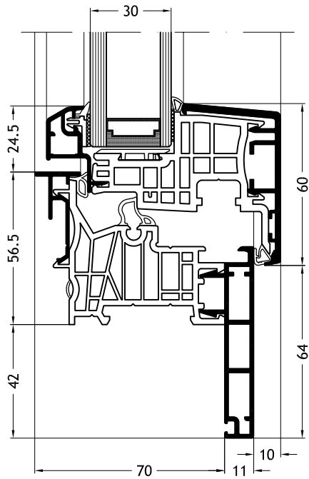
Blendrahmen Z-Form D2X mit Flügel Classic-line A26
