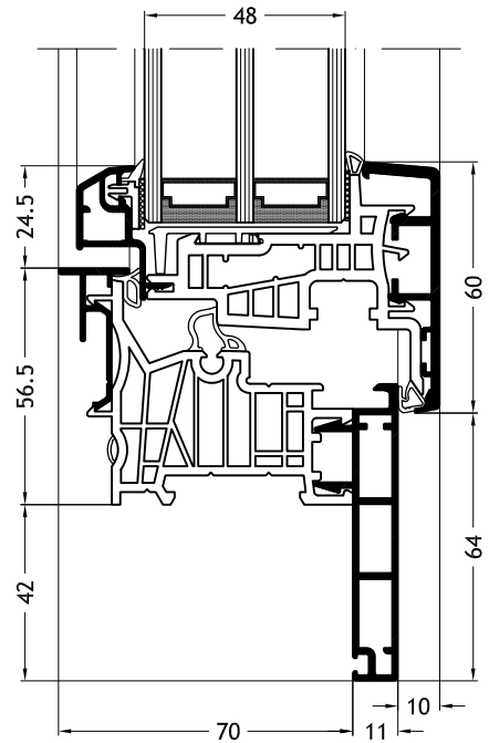
Blendrahmen Z-Form D2X mit Flügel Classic-line A27
