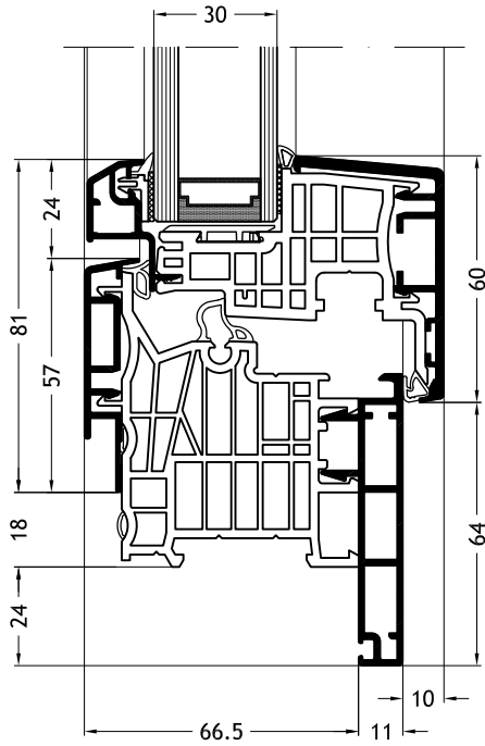
Blendrahmen L-Form D1Y mit Flügel Classic-line A26
