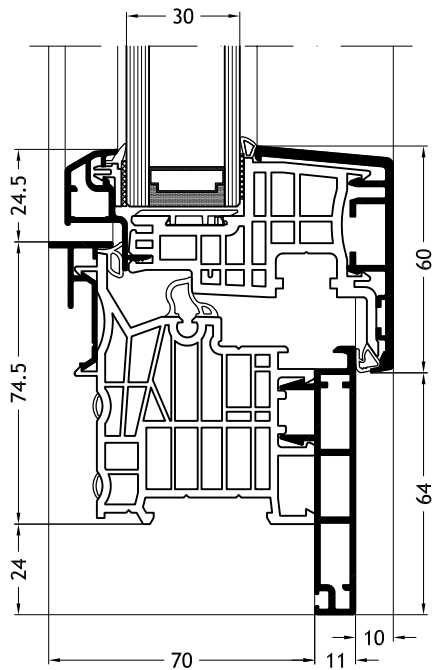
Blendrahmen L-Form D1X mit Flügel Classic-line A26
