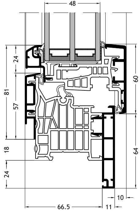
Blendrahmen L-Form D1Y mit Flügel Classic-line A27
