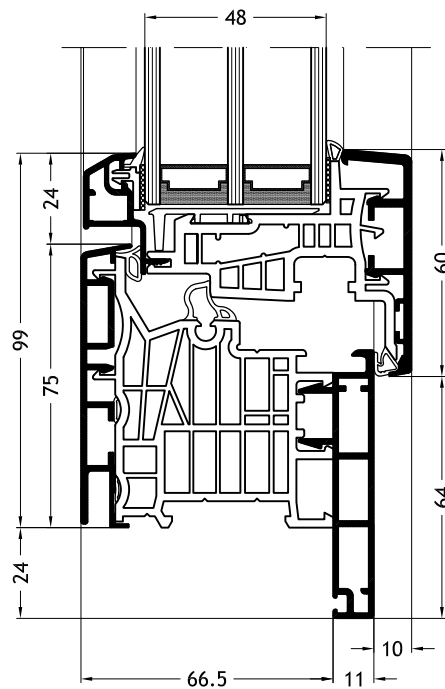
Blendrahmen L-Form D1W mit Flügel Classic-line A27
