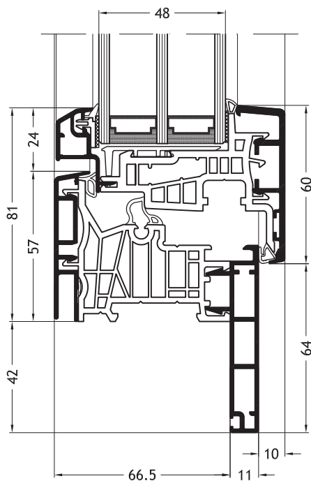
Telaio a Z D2Y con anta Classic-line A27
