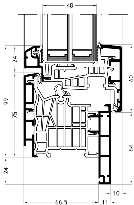
Telaio a L D1Z con anta Classic-line A27
