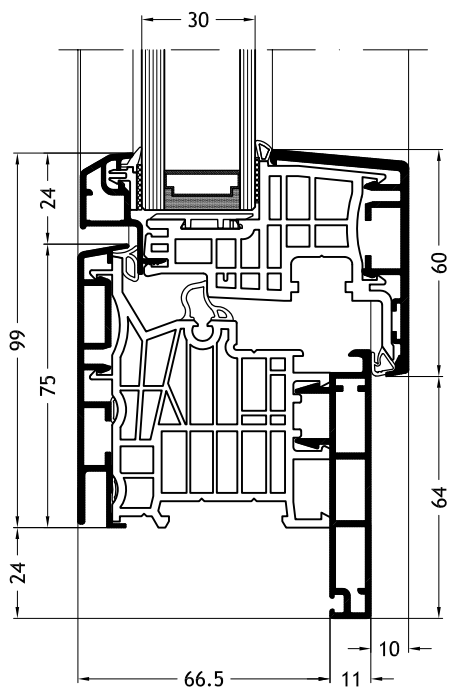
Telaio a L D1W con anta Classic-line A26
