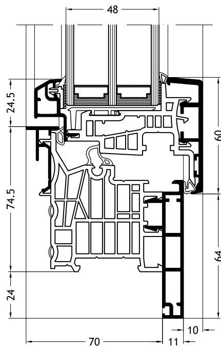
Telaio a L D1X con anta Classic-line A27
