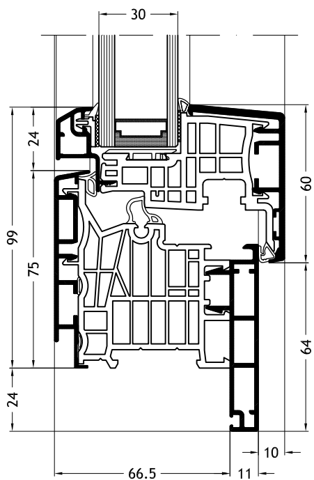
Telaio a L D1Z con anta Classic-line A26
