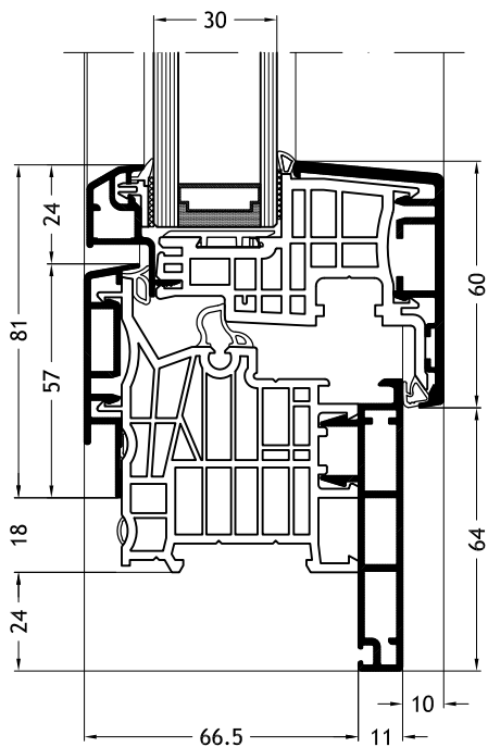
Telaio a L D1Y con anta Classic-line A26
