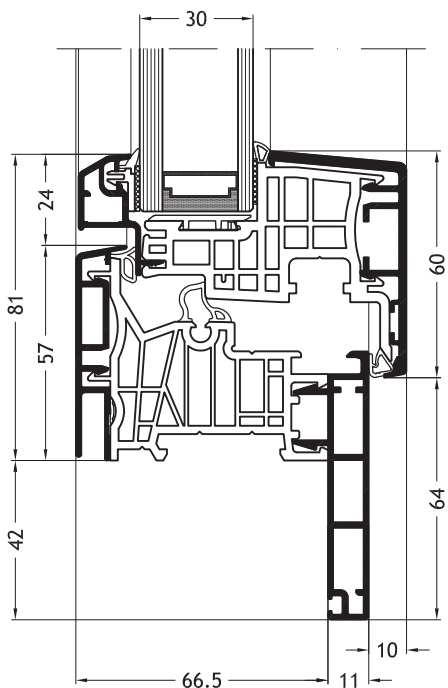
Telaio a Z D2Y con anta Classic-line A26
