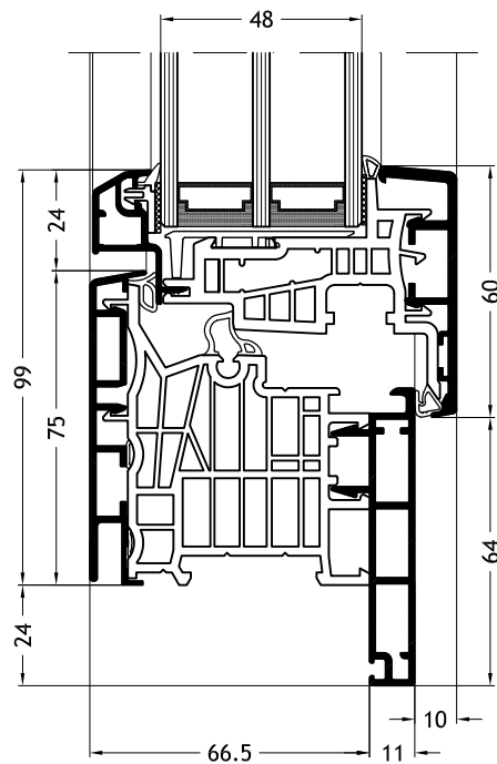
Telaio a L D1W con anta Classic-line A27
