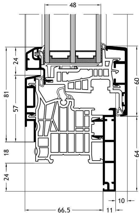
Telaio a L D1Y con anta Classic-line A27
