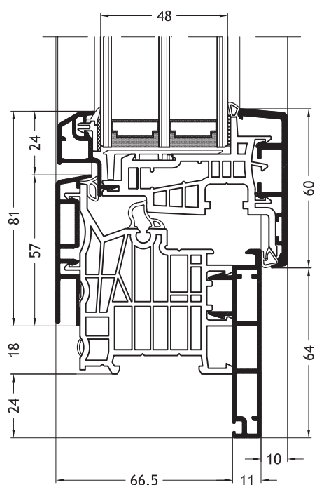
Telaio a L D1V con anta Classic-line A27
