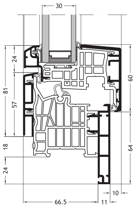
Telaio a L D1V con anta Classic-line A26
