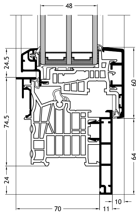
Dormant en L, D1X avec ouvrant Classic-line A27
