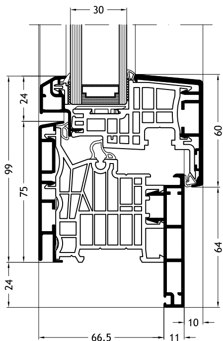
Dormant en L, D1W avec ouvrant Classic-line A26
