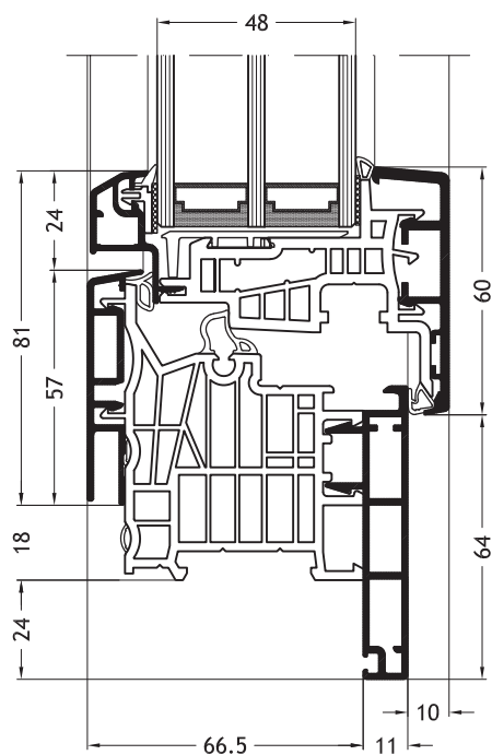
Dormant en L, D1V avec ouvrant Classic-line A27
