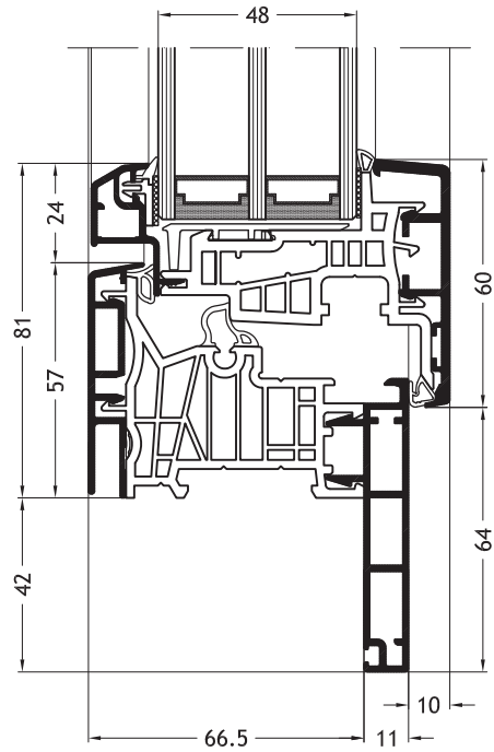
Dormant en Z, D2Y avec ouvrant Classic-line A27
