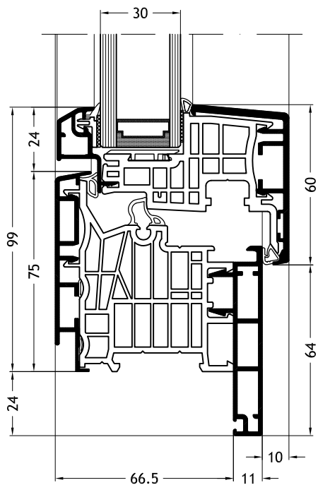
Dormant en L, D1Z avec ouvrant Classic-line A26
