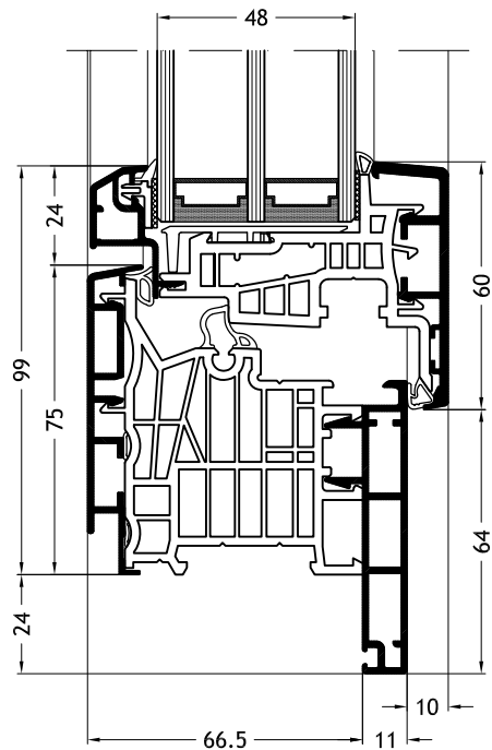
Dormant en L, D1Z avec ouvrant Classic-line A27
