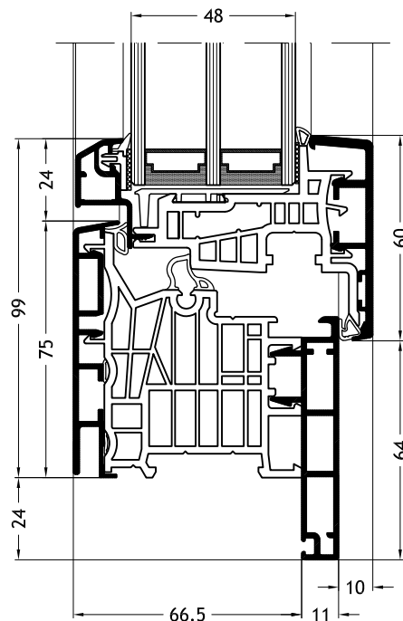
Dormant en L, D1W avec ouvrant Classic-line A27
