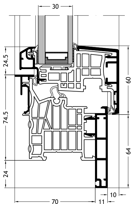
Dormant en L, D1X avec ouvrant Classic-line A26
