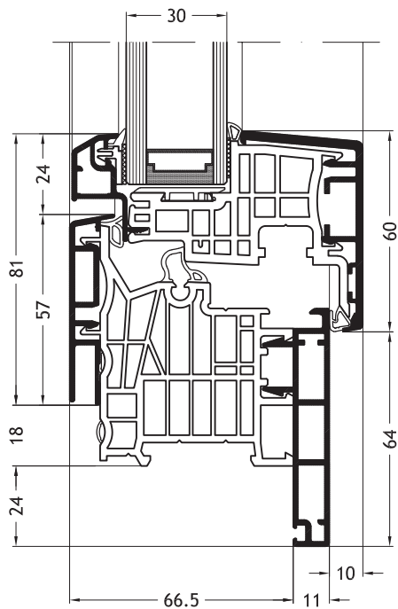
Dormant en L, D1V avec ouvrant Classic-line A26
