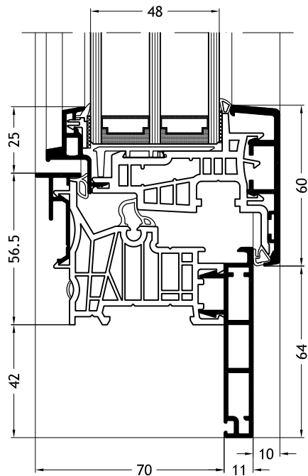
Blendrahmen Z-Form D2X mit Flügel Ferro-line A18
