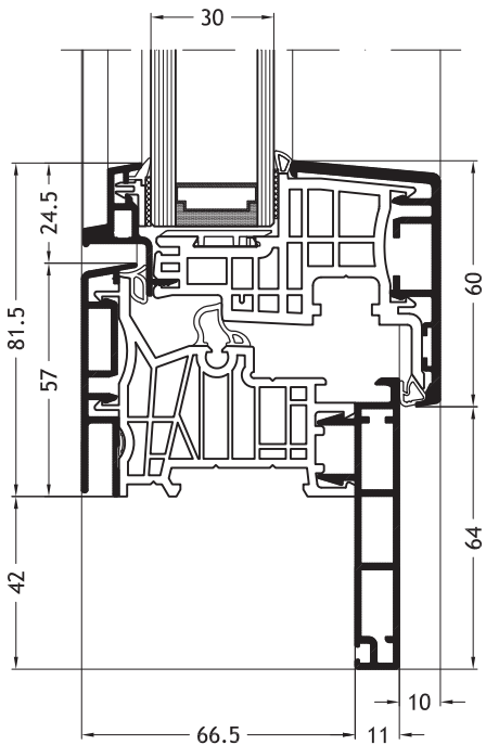
Blendrahmen Z-Form D2V mit Flügel Ferro-line A14
