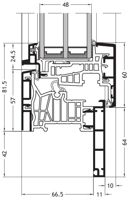
Blendrahmen Z-Form D2V mit Flügel Ferro-line A18
