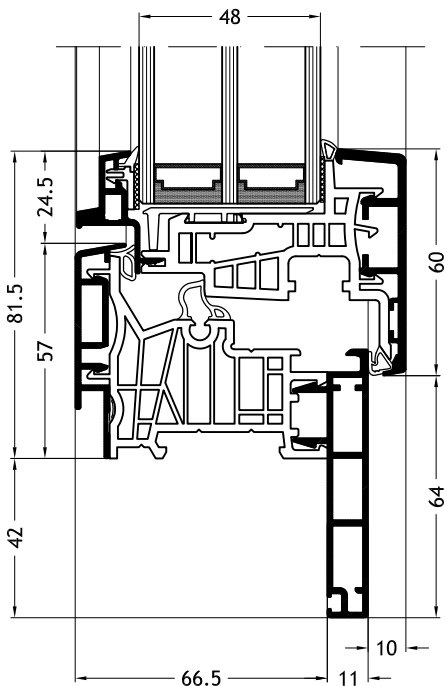
Blendrahmen Z-Form D2Y mit Flügel Ferro-line A18
