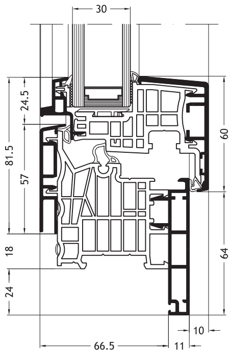
Blendrahmen L-Form D1V mit Flügel Ferro-line A14
