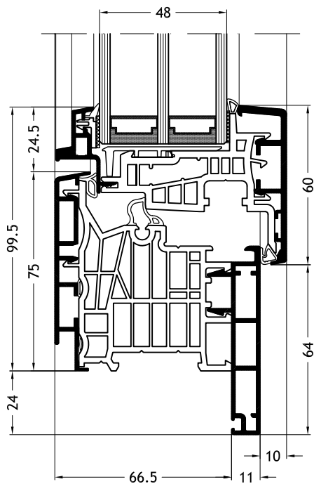
Blendrahmen L-Form D1Z mit Flügel Ferro-line A18
