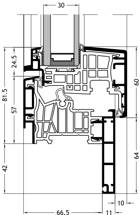
Blendrahmen Z-Form D2Y mit Flügel Ferro-line A14
