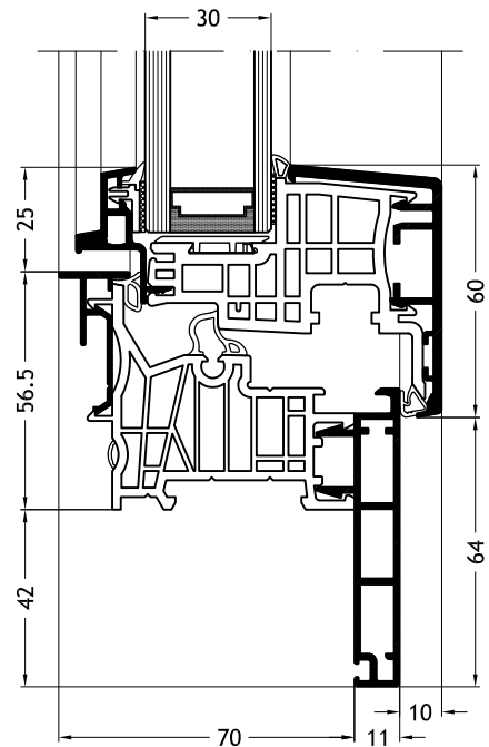
Blendrahmen Z-Form D2X mit Flügel Ferro-line A14
