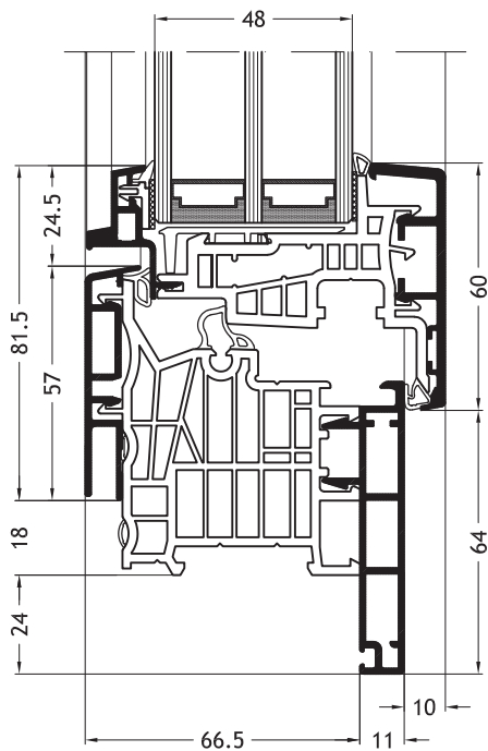
Blendrahmen L-Form D1V mit Flügel Ferro-line A18
