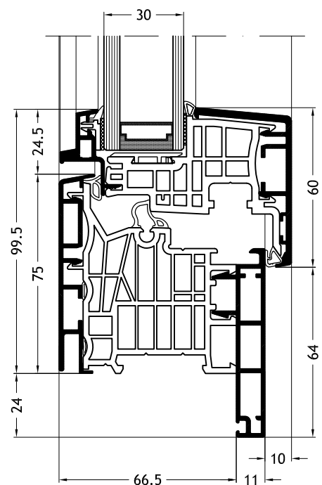
Blendrahmen L-Form D1W mit Flügel Ferro-line A14
