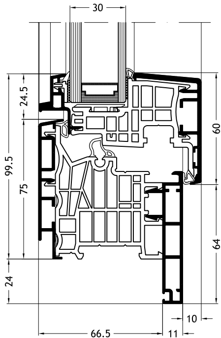
Blendrahmen L-Form D1Z mit Flügel Ferro-line A14
