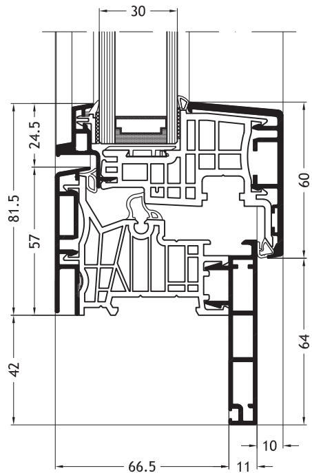
Dormant en Z, D2V avec ouvrant Ferro-line A14
