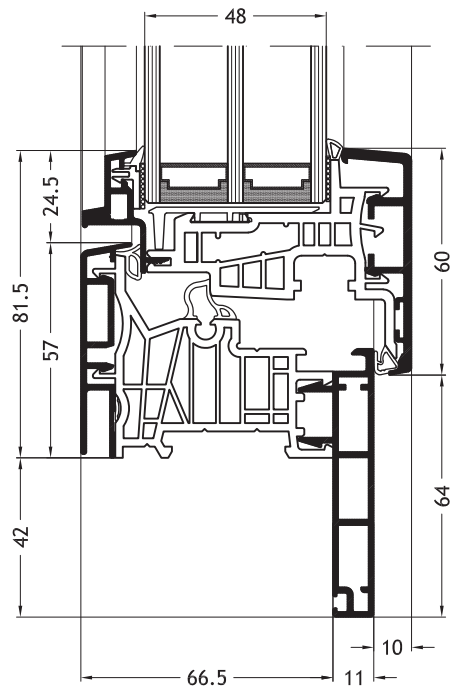
Dormant en Z, D2V avec ouvrant Ferro-line A18
