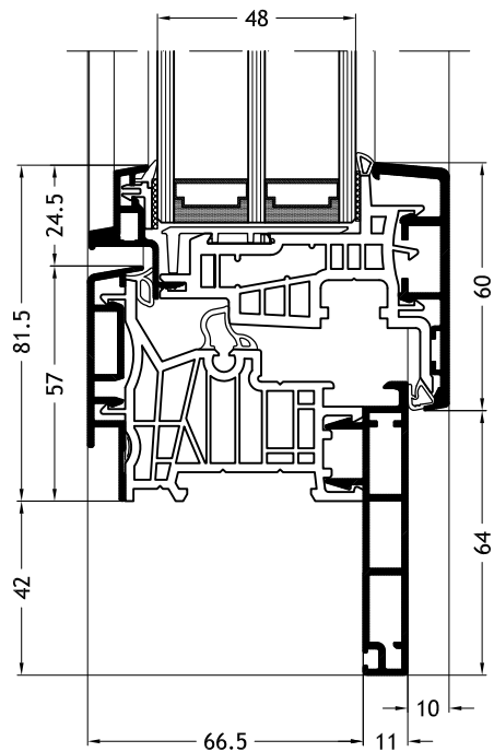
Dormant en Z, D2Y avec ouvrant Ferro-line A18
