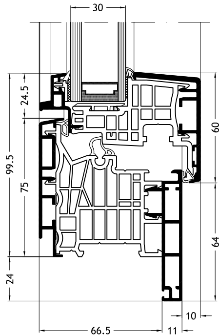
Dormant en L, D1Z avec ouvrant Ferro-line A14
