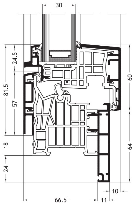
Dormant en L, D1V avec ouvrant Ferro-line A14
