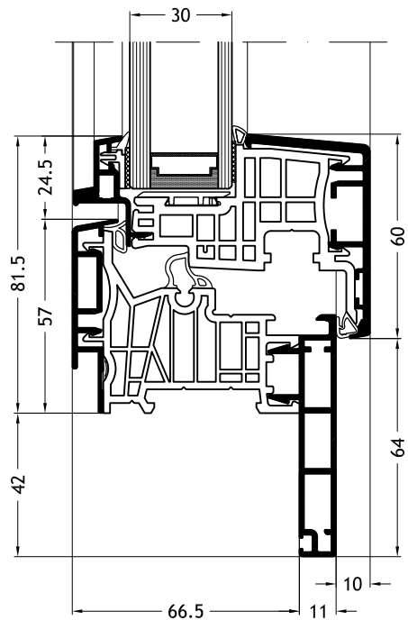
Dormant en Z, D2Y avec ouvrant Ferro-line A14
