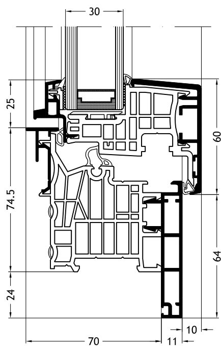
Kozijn L-vorm D1X met vleugel Ferro-line A14
