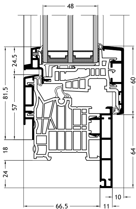
Kozijn L-vorm D1Y met vleugel Ferro-line A18
