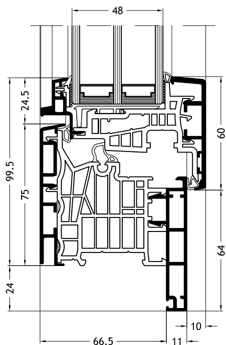
Kozijn L-vorm D1W met vleugel Ferro-line A18
