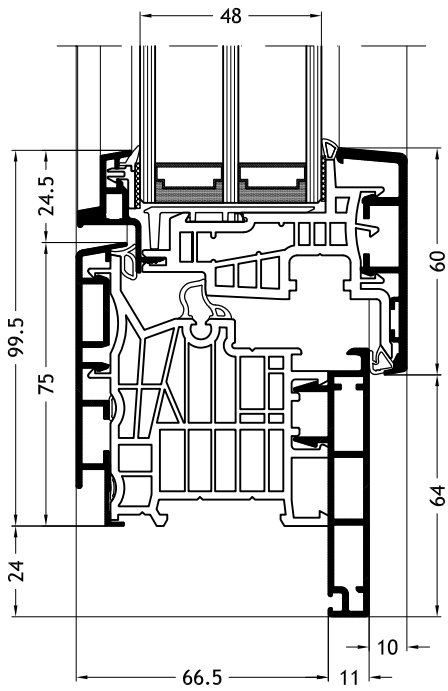
Kozijn L-vorm D1Z met vleugel Ferro-line A18
