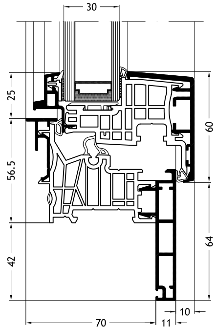
Kozijn Z-vorm D2X met vleugel Ferro-line A14
