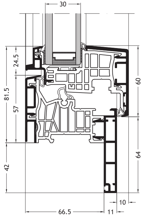
Kozijn Z-vorm D2V met vleugel Ferro-line A14
