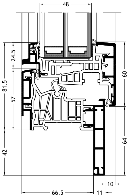
Kozijn Z-vorm D2Y met vleugel Ferro-line A18
