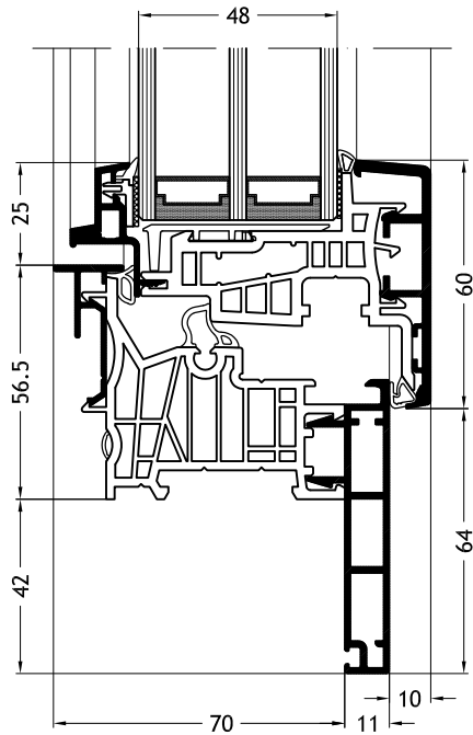
Kozijn Z-vorm D2X met vleugel Ferro-line A18
