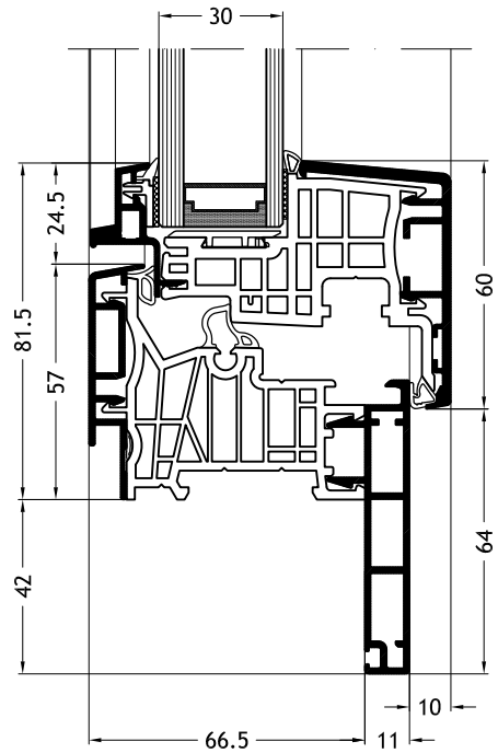
Kozijn Z-vorm D2Y met vleugel Ferro-line A14
