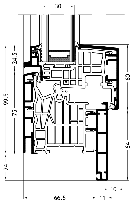
Kozijn L-vorm D1W met vleugel Ferro-line A14
