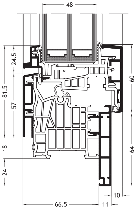
Kozijn L-vorm D1V met vleugel Ferro-line A18
