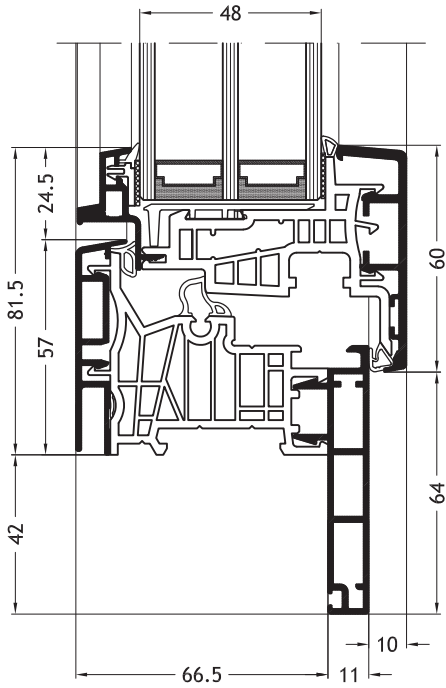
Kozijn Z-vorm D2V met vleugel Ferro-line A18
