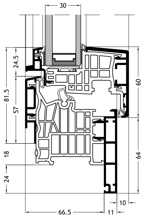
Kozijn L-vorm D1Y met vleugel Ferro-line A14
