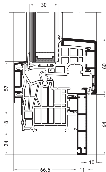
Blendrahmen L-Form D1Y mit Flügel Nova-line A10
