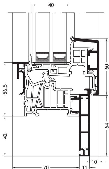
Blendrahmen Z-Form D2X mit Flügel Nova-line A11
