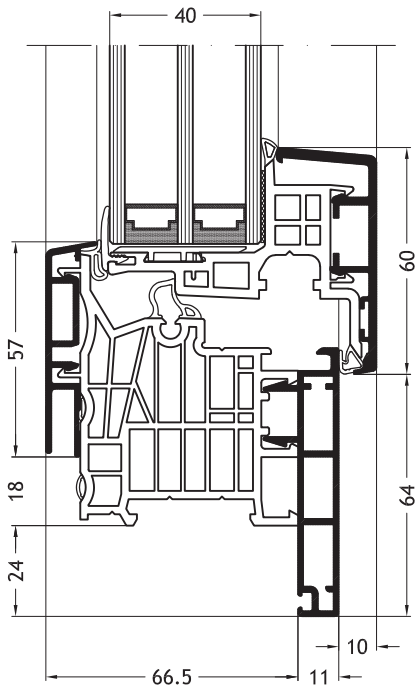
Blendrahmen L-Form D1V mit Flügel Nova-line A11
