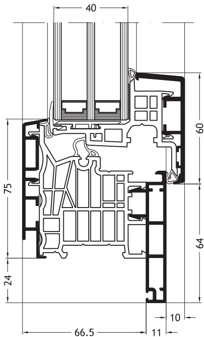
Blendrahmen L-Form D1Z mit Flügel Nova-line A11
