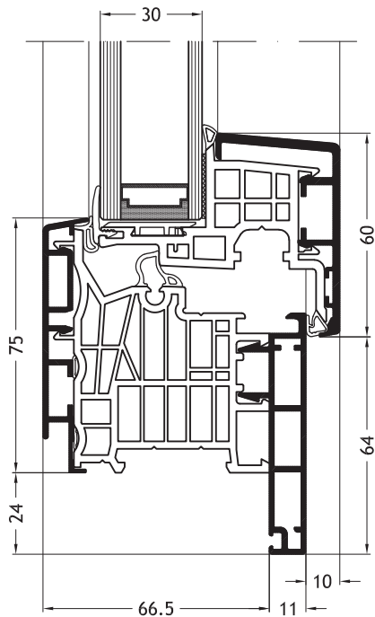
Blendrahmen L-Form D1Z mit Flügel Nova-line A10
