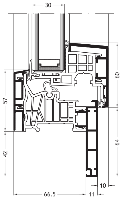
Blendrahmen Z-Form D2V mit Flügel Nova-line A10
