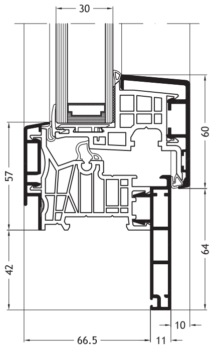
Blendrahmen Z-Form D2Y mit Flügel Nova-line A10
