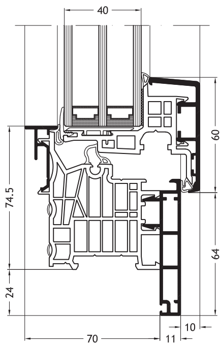
Blendrahmen L-Form D1X mit Flügel Nova-line A11
