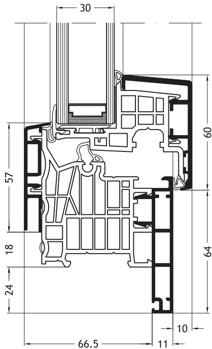
Blendrahmen L-Form D1V mit Flügel Nova-line A10
