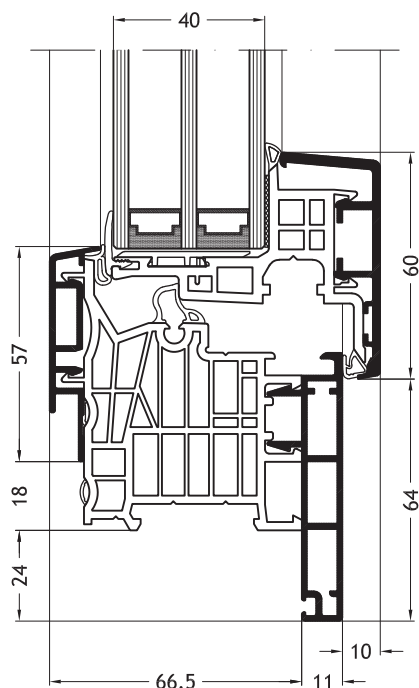
Blendrahmen L-Form D1Y mit Flügel Nova-line A11
