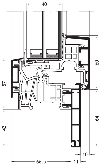
Blendrahmen Z-Form D2Y mit Flügel Nova-line A11
