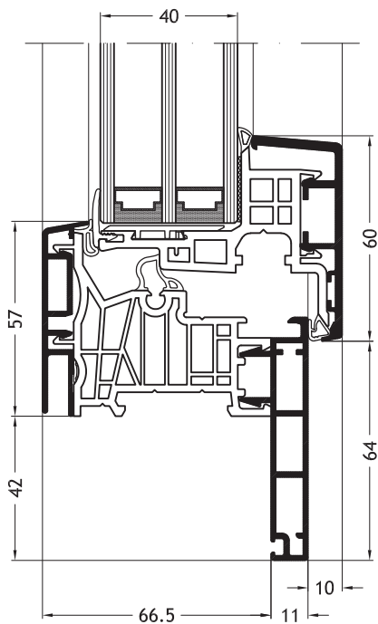
Blendrahmen Z-Form D2V mit Flügel Nova-line A11
