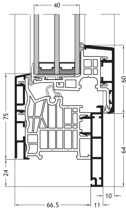
Blendrahmen L-Form D1W mit Flügel Nova-line A11
