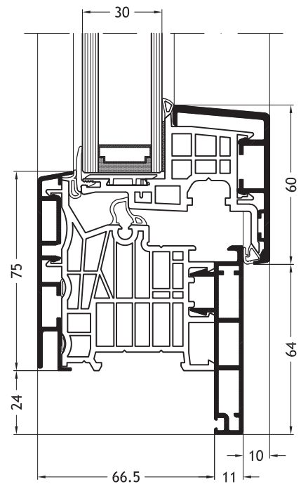
Blendrahmen L-Form D1W mit Flügel Nova-line A10
