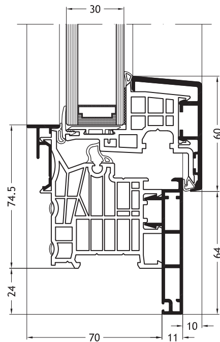
Blendrahmen L-Form D1X mit Flügel Nova-line A10
