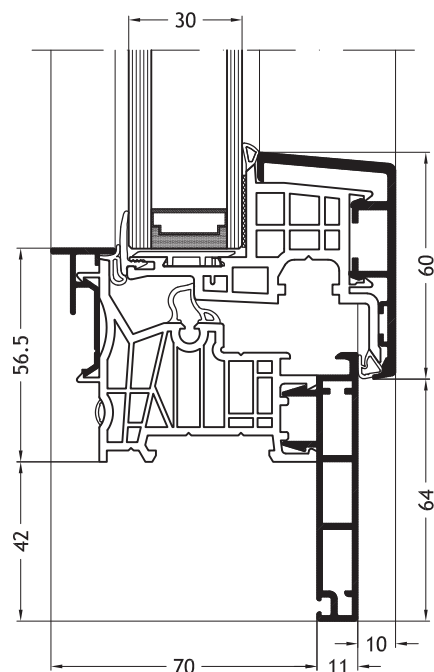
Blendrahmen Z-Form D2X mit Flügel Nova-line A10
