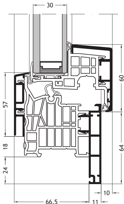
Aro em forma de L D1V com folha Nova-line A10
