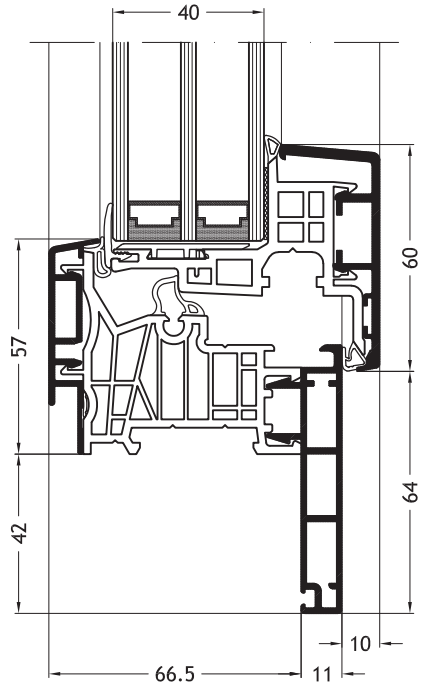
Aro em forma de Z D2Y com folha Nova-line A11
