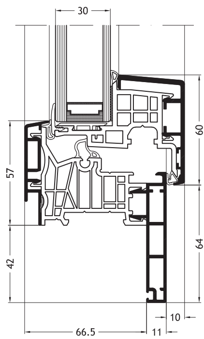
Aro em forma de Z D2Y com folha Nova-line A10
