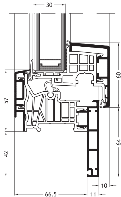
Telaio a Z D2Y con anta Nova-line A10
