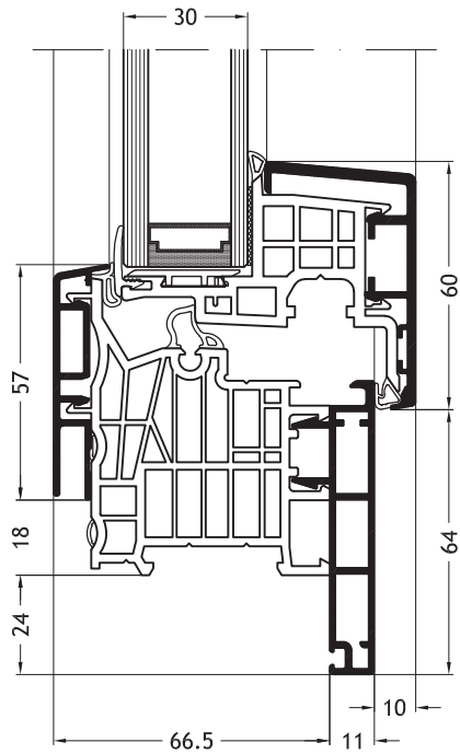
Telaio a L D1V con anta Nova-line A10
