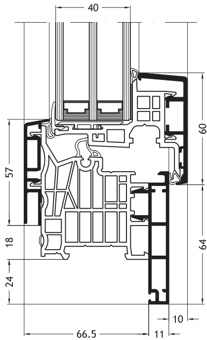
Telaio a L D1V con anta Nova-line A11
