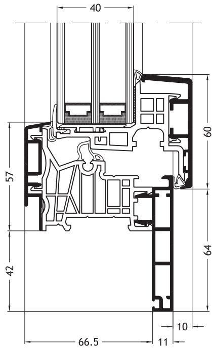
Telaio a Z D2Y con anta Nova-line A11
