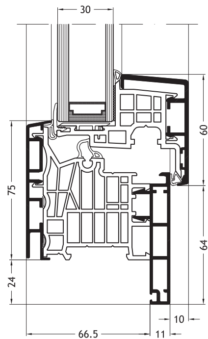
Telaio a L D1W con anta Nova-line A10
