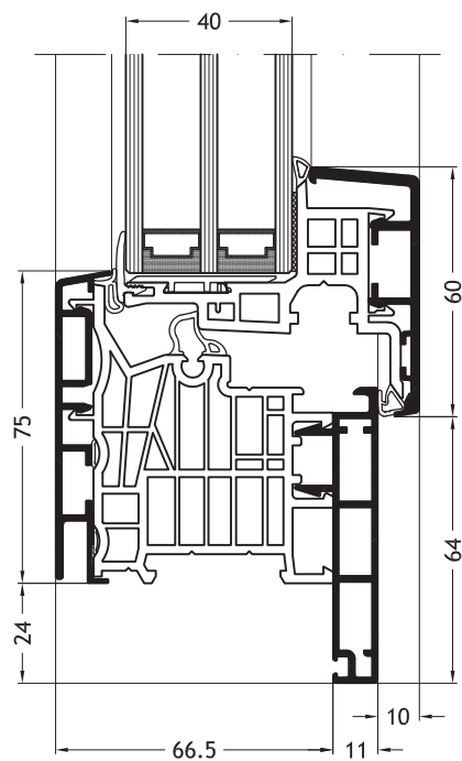
Telaio a L D1W con anta Nova-line A11
