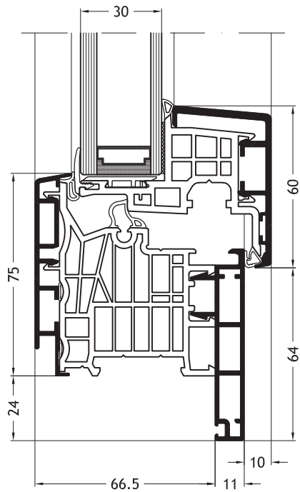
Telaio a L D1Z con anta Nova-line A10
