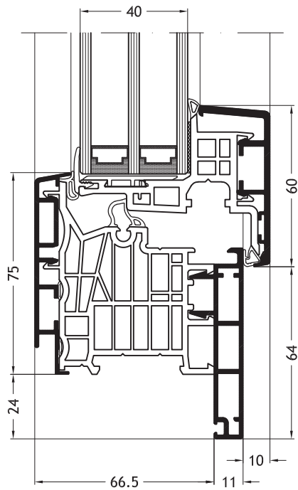
Telaio a L D1Z con anta Nova-line A11
