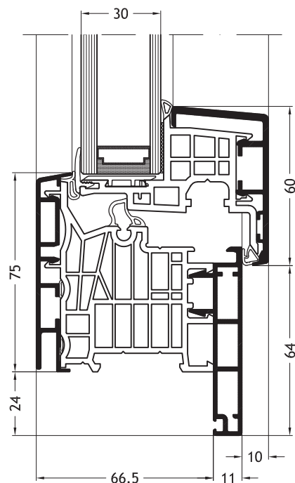
Dormant en L, D1W avec ouvrant Nova-line A10
