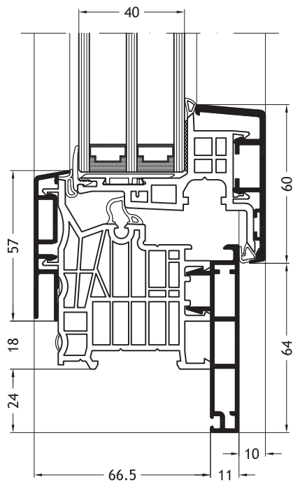
Dormant en L, D1V avec ouvrant Nova-line A11
