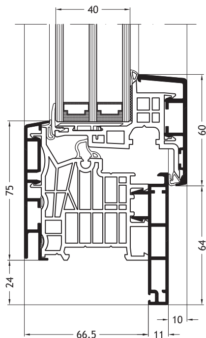
Dormant en L, D1W avec ouvrant Nova-line A11
