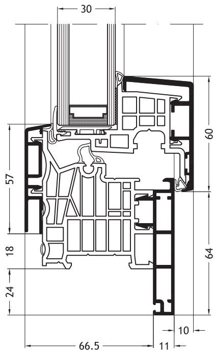
Dormant en L, D1V avec ouvrant Nova-line A10
