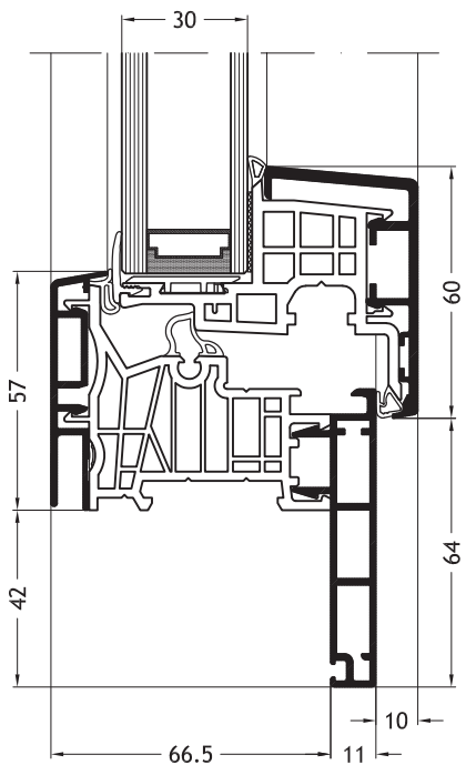
Dormant en Z, D2V avec ouvrant Nova-line A10
