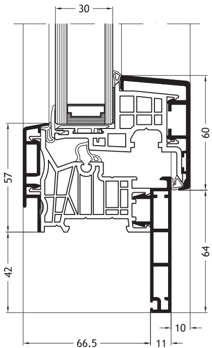
Dormant en Z, D2Y avec ouvrant Nova-line A10
