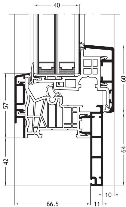
Dormant en Z, D2Y avec ouvrant Nova-line A11
