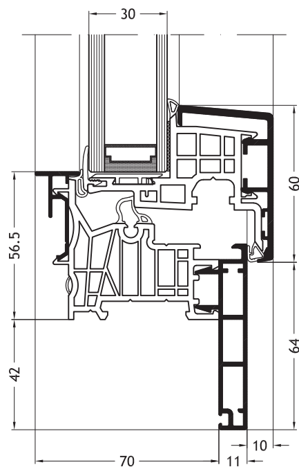
Kozijn Z-vorm D2X met vleuge Nova-line A10
