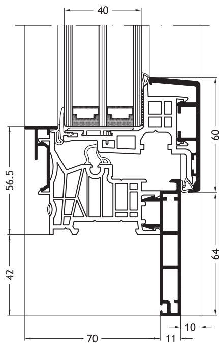
Kozijn Z-vorm D2X met vleuge Nova-line A11
