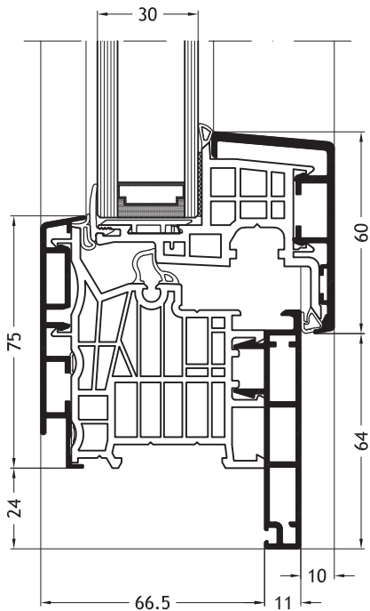
Kozijn L-vorm D1Z met vleuge Nova-line A10
