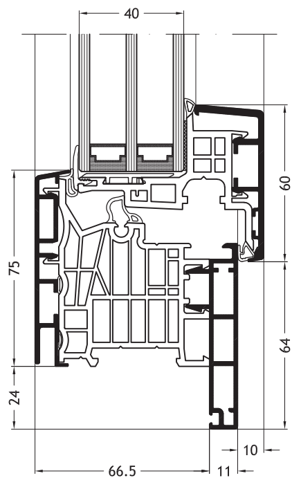
Kozijn L-vorm D1W met vleuge Nova-line A11
