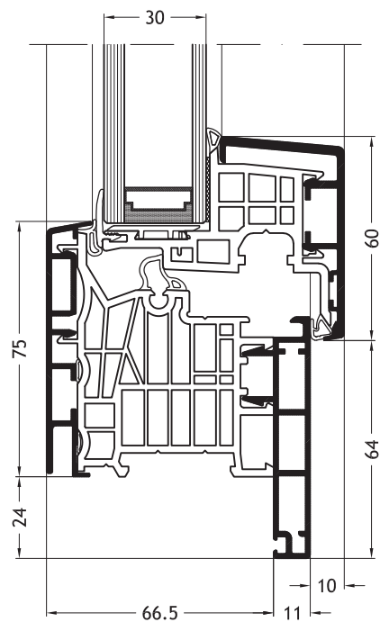
Kozijn L-vorm D1W met vleuge Nova-line A10
