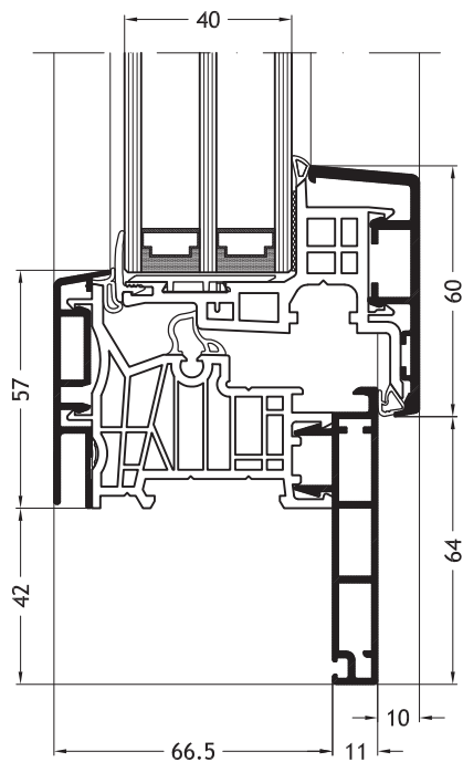
Kozijn Z-vorm D2V met vleuge Nova-line A11
