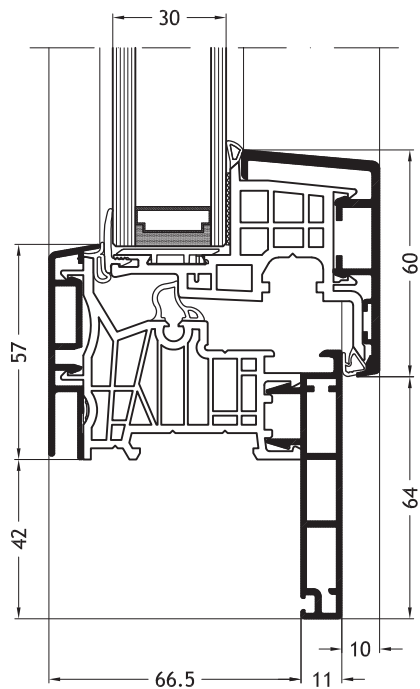
Kozijn Z-vorm D2V met vleuge Nova-line A10
