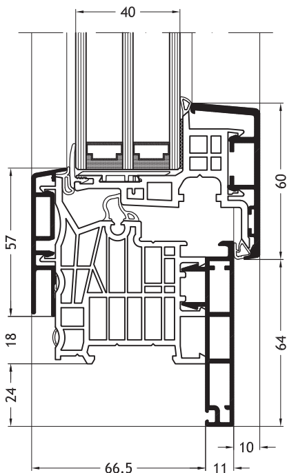
Kozijn L-vorm D1V met vleuge Nova-line A11
