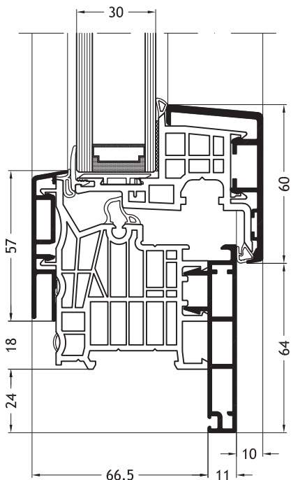
Kozijn L-vorm D1V met vleuge Nova-line A10
