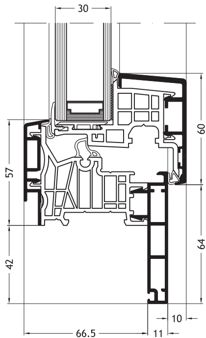
Kozijn Z-vorm D2Y met vleuge Nova-line A10
