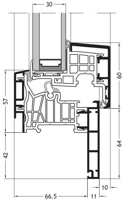
Frame Z-vorm D2Y met vleugel Nova-line A10
