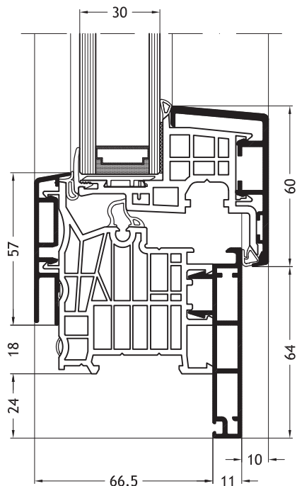
Frame L-vorm D1V met vleugel Nova-line A10
