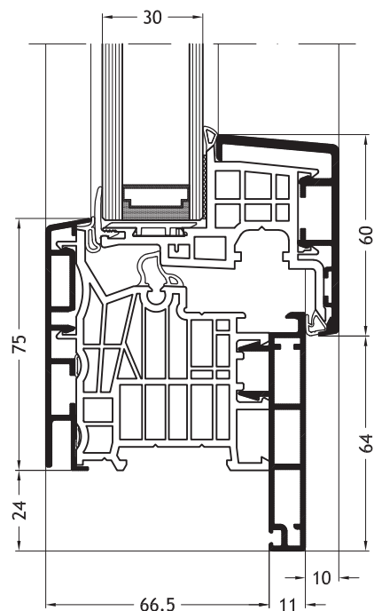
Frame L-vorm D1W met vleugel Nova-line A10
