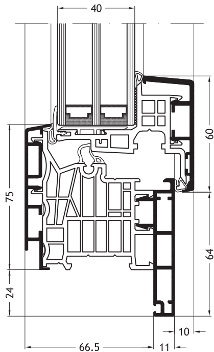
Frame L-vorm D1Z met vleugel Nova-line A11
