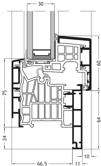
Frame L-vorm D1Z met vleugel Nova-line A10
