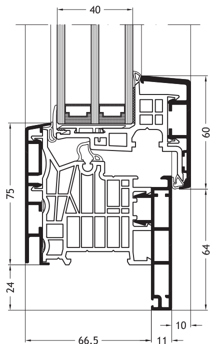
Frame L-vorm D1W met vleugel Nova-line A11
