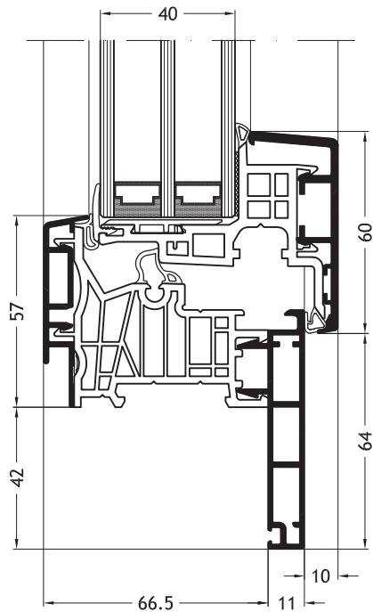
Frame Z-vorm D2Y met vleugel Nova-line A11
