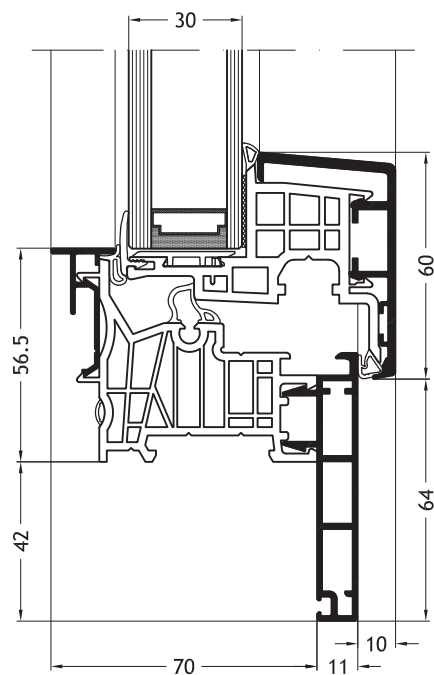
Frame Z-vorm D2X met vleugel Nova-line A10
