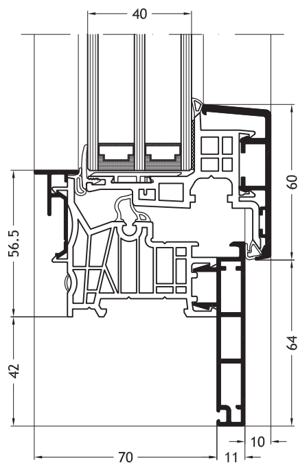
Frame Z-vorm D2X met vleugel Nova-line A11
