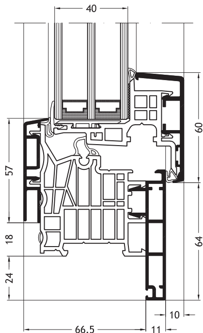
Frame L-vorm D1V met vleugel Nova-line A11
