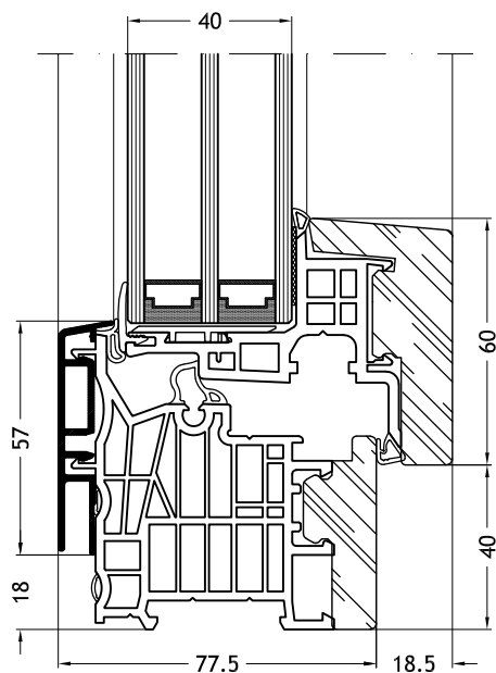
Dormant en L, 9A1V avec ouvrant Nova-line 9A11
