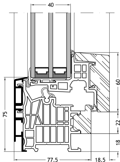
Dormant en L, 9C1Z avec ouvrant Nova-line 9A11
