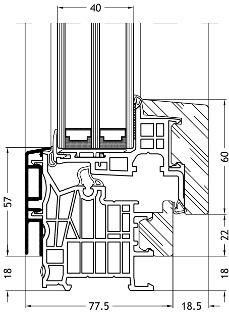
Dormant en L, 9C1V avec ouvrant Nova-line 9A11
