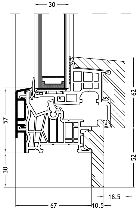
Dormant en Z, 9B2Y avec ouvrant Nova-line 9A10
