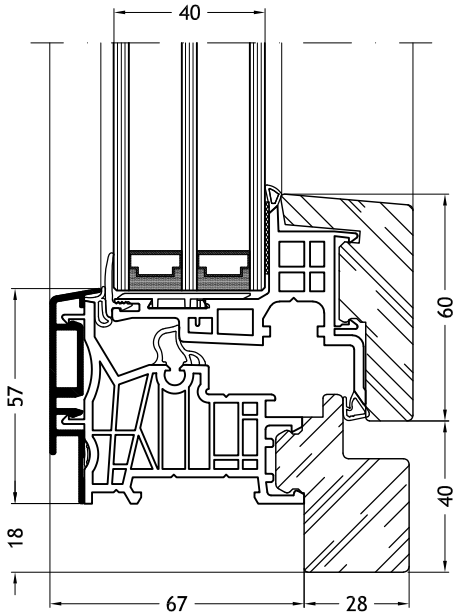
Dormant en Z, 9F2Y avec ouvrant Nova-line 9A11
