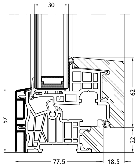
Dormant en Z, 9C2V avec ouvrant Nova-line 9A10
