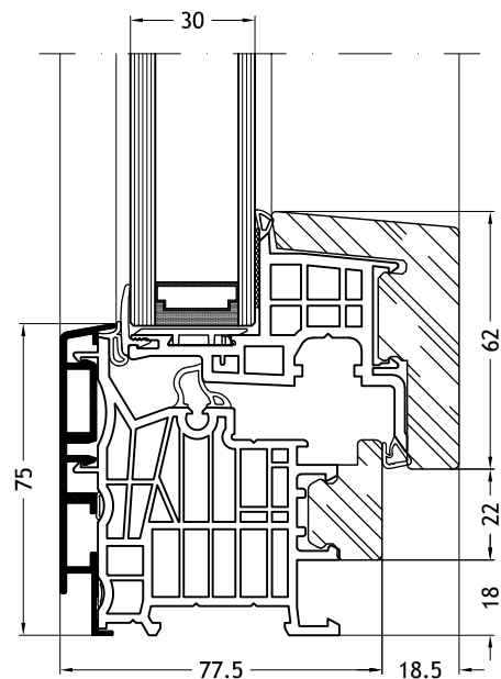
Dormant en L, 9C1Z avec ouvrant Nova-line 9A10
