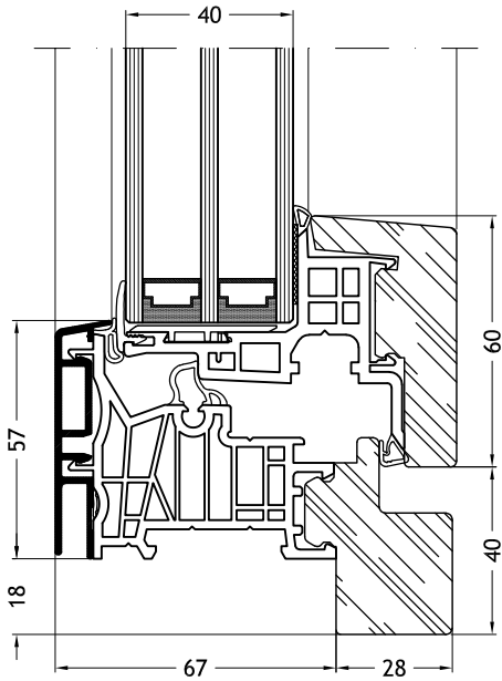
Dormant en Z, 9F2V avec ouvrant Nova-line 9A11
