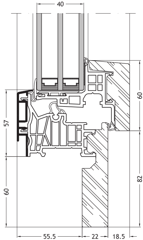
Dormant en Z, 9H2V avec ouvrant Nova-line 9A11
