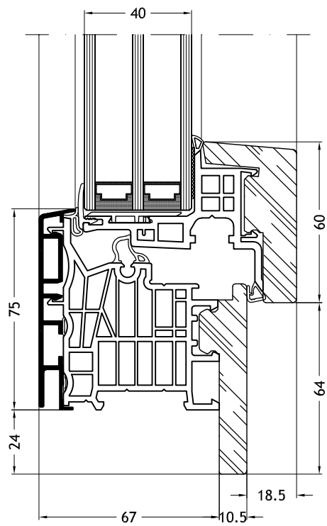
Dormant en L, 9D1W avec ouvrant Nova-line 9A11
