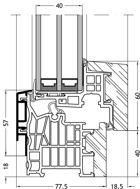
Dormant en L, 9A1Y avec ouvrant Nova-line 9A11
