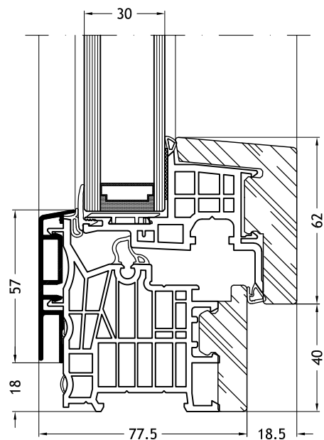
Dormant en L, 9A1V avec ouvrant Nova-line 9A10
