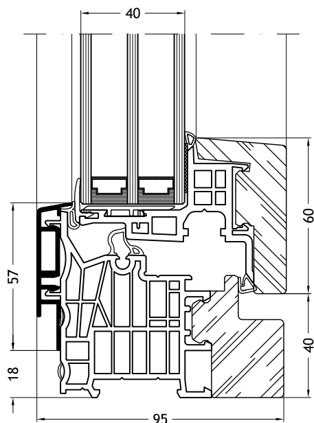
Dormant en L, 9F1Y avec ouvrant Nova-line 9A11
