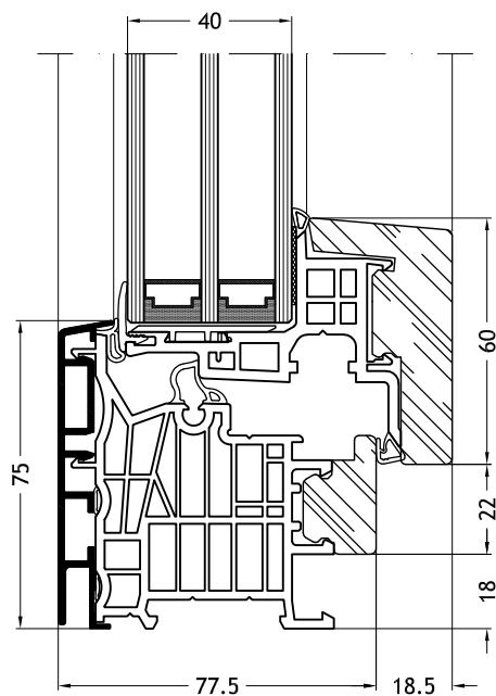
Dormant en L, 9C1W avec ouvrant Nova-line 9A11
