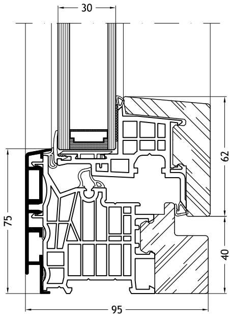
Dormant en L, 9F1Z avec ouvrant Nova-line 9A10
