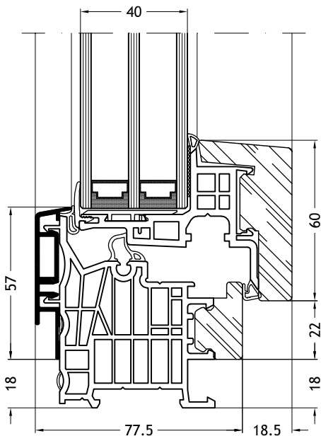
Dormant en L, 9C1Y avec ouvrant Nova-line 9A11
