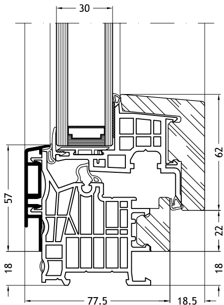
Dormant en L, 9C1Y avec ouvrant Nova-line 9A10
