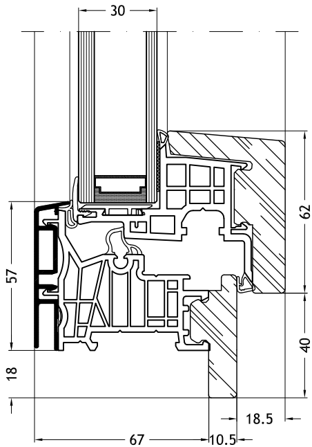
Dormant en Z, 9A2V avec ouvrant Nova-line 9A10
