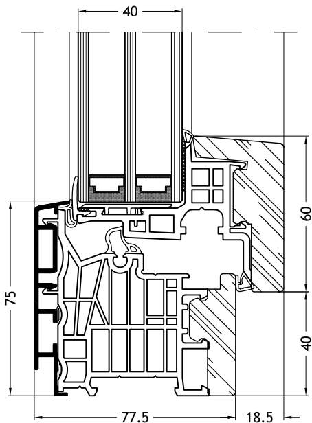
Dormant en L, 9A1Z avec ouvrant Nova-line 9A11
