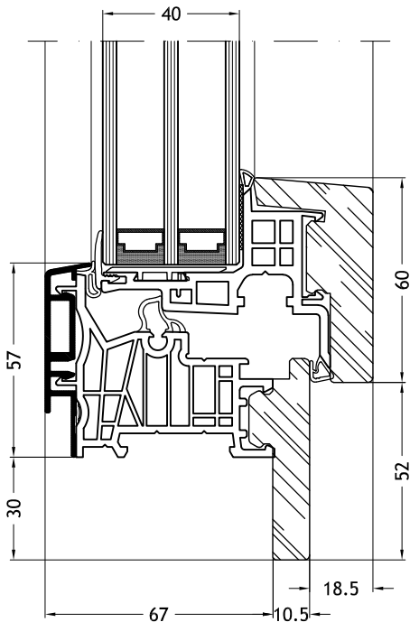
Dormant en Z, 9B2Y avec ouvrant Nova-line 9A11
