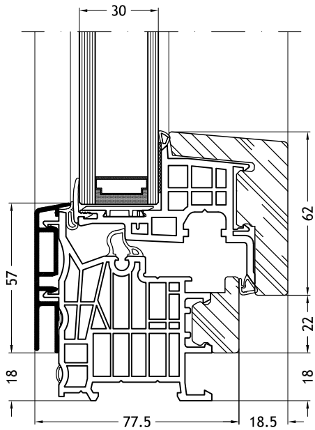
Dormant en L, 9C1V avec ouvrant Nova-line 9A10
