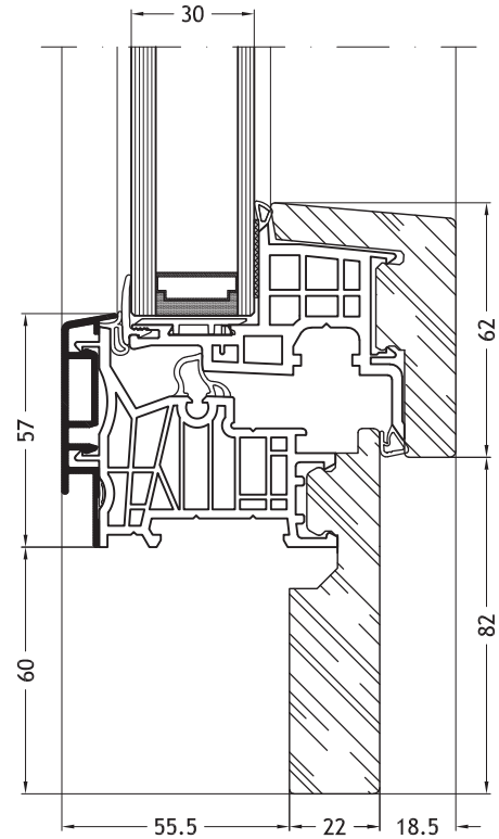
Dormant en Z, 9H2V avec ouvrant Nova-line 9A10
