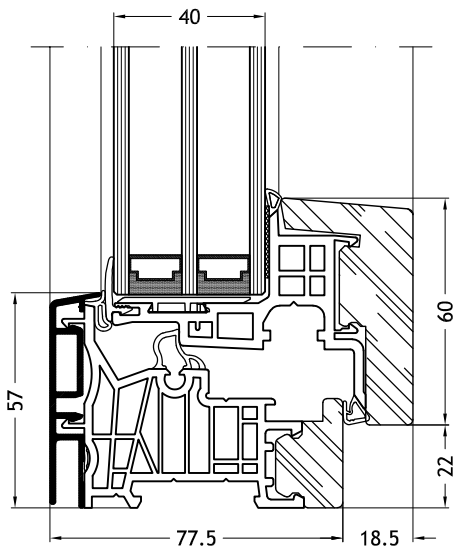
Dormant en Z, 9C2V avec ouvrant Nova-line 9A11
