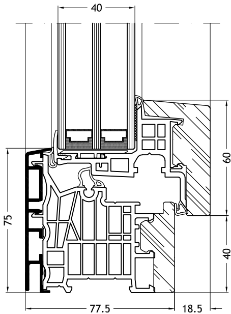
Dormant en L, 9A1W avec ouvrant Nova-line 9A11
