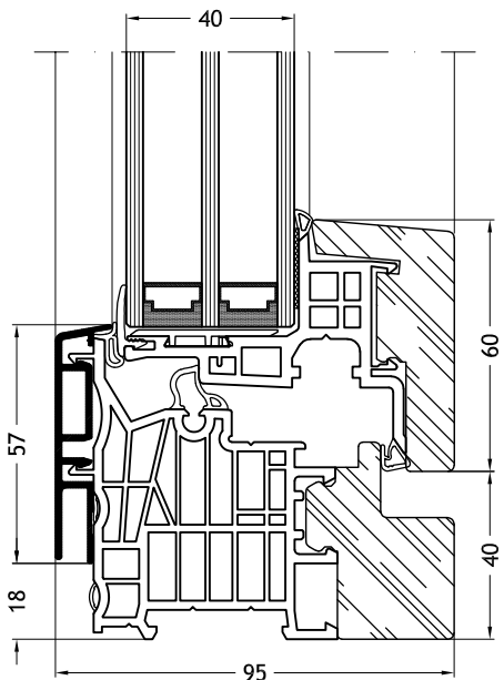
Dormant en L, 9F1V avec ouvrant Nova-line 9A11
