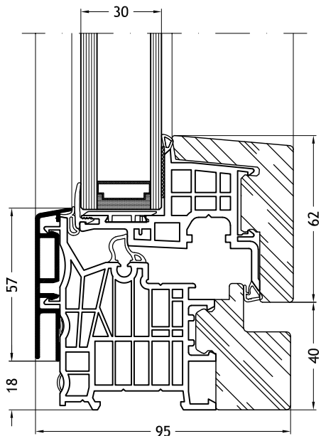
Dormant en L, 9F1V avec ouvrant Nova-line 9A10
