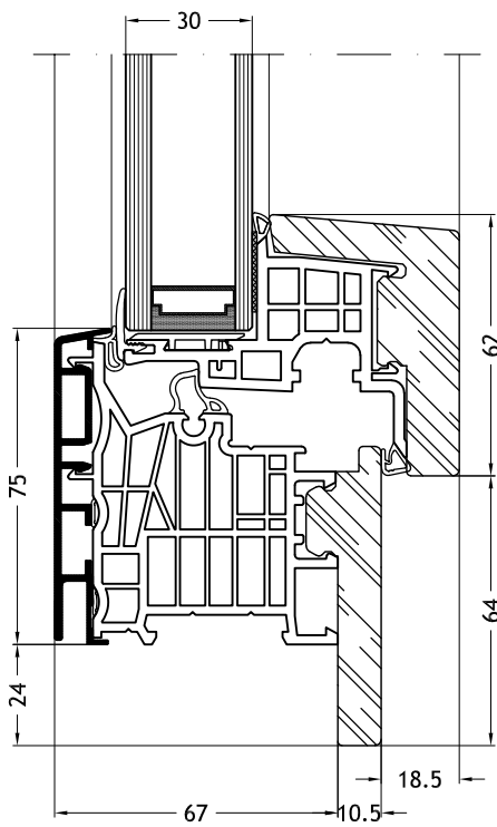
Dormant en L, 9D1W avec ouvrant Nova-line 9A10
