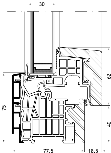
Dormant en L, 9A1Z avec ouvrant Nova-line 9A10
