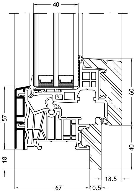
Dormant en Z, 9A2V avec ouvrant Nova-line 9A11
