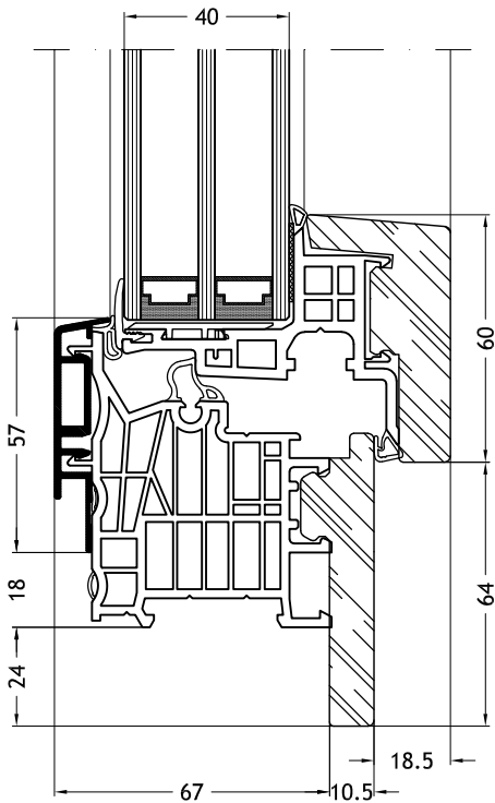
Dormant en L, 9D1Y avec ouvrant Nova-line 9A11
