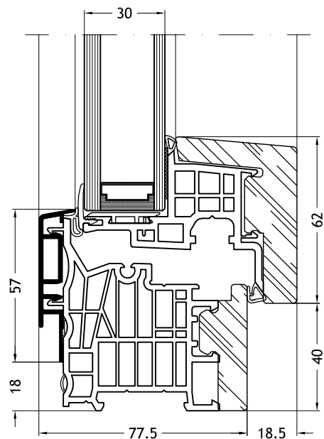
Dormant en L, 9A1Y avec ouvrant Nova-line 9A10
