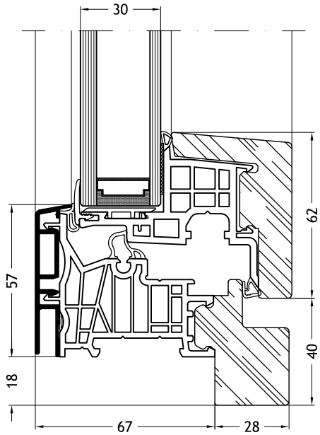
Dormant en Z, 9F2V avec ouvrant Nova-line 9A10
