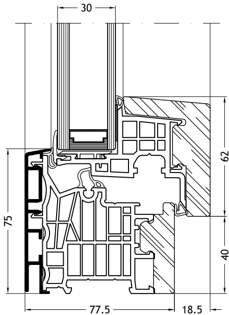
Dormant en L, 9A1W avec ouvrant Nova-line 9A10
