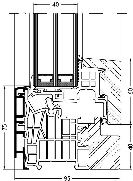
Dormant en L, 9F1Z avec ouvrant Nova-line 9A11
