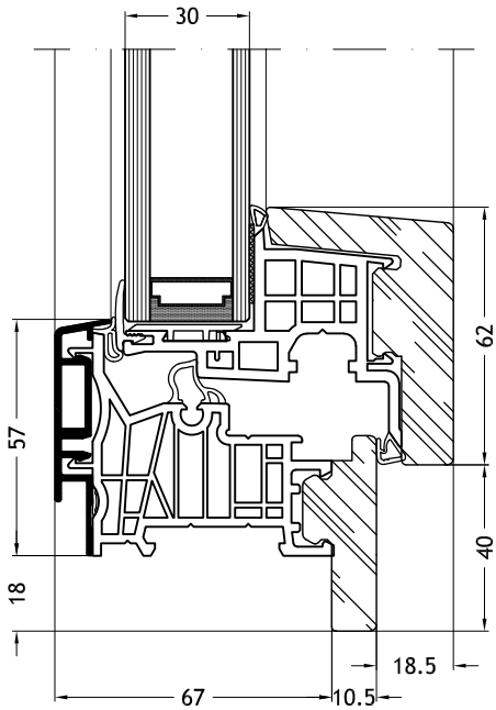
Dormant en Z, 9A2Y avec ouvrant Nova-line 9A10
