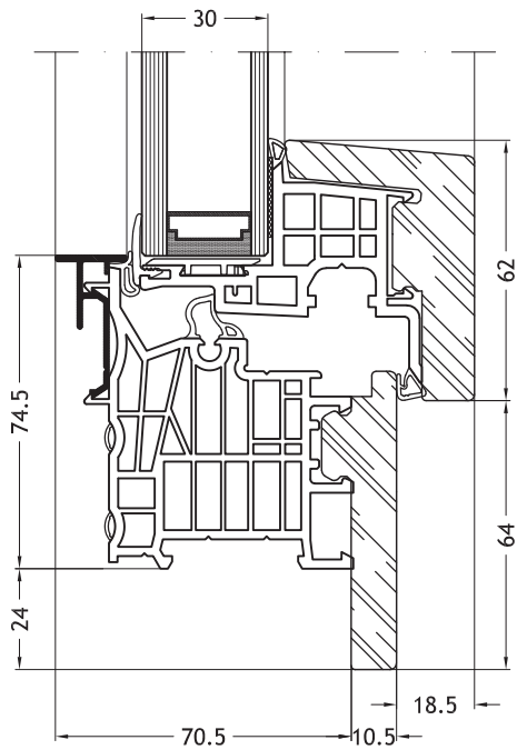
Dormant en L, 9D1X avec ouvrant Nova-line 9A10
