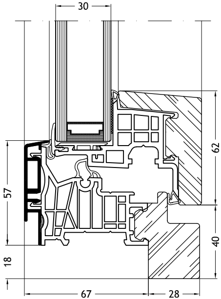
Dormant en Z, 9F2Y avec ouvrant Nova-line 9A10
