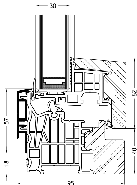
Dormant en L, 9F1Y avec ouvrant Nova-line 9A10
