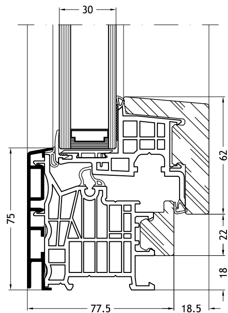
Dormant en L, 9C1W avec ouvrant Nova-line 9A10
