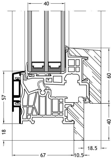
Dormant en Z, 9A2Y avec ouvrant Nova-line 9A11
