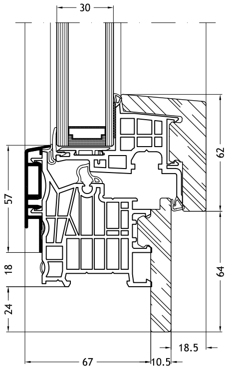
Dormant en L, 9D1Y avec ouvrant Nova-line 9A10
