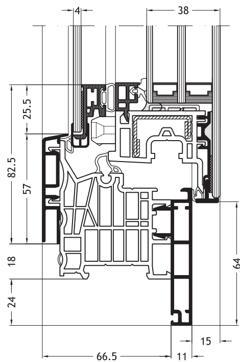
Blendrahmen L-Form D1V mit Flügel Nova-line Cristal Twin A34
