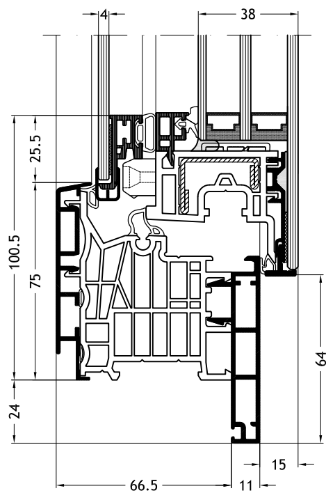
Blendrahmen L-Form D1Z mit Flügel Nova-line Cristal Twin A34
