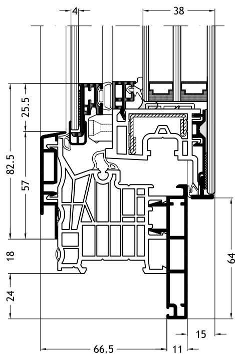
Blendrahmen L-Form D1Y mit Flügel Nova-line Cristal Twin A34
