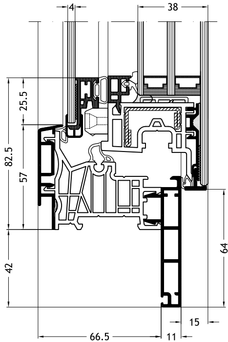
Blendrahmen Z-Form D2Y mit Flügel Nova-line Cristal Twin A34
