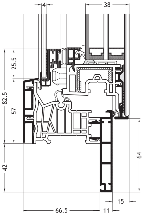
Blendrahmen Z-Form D2V mit Flügel Nova-line Cristal Twin A34
