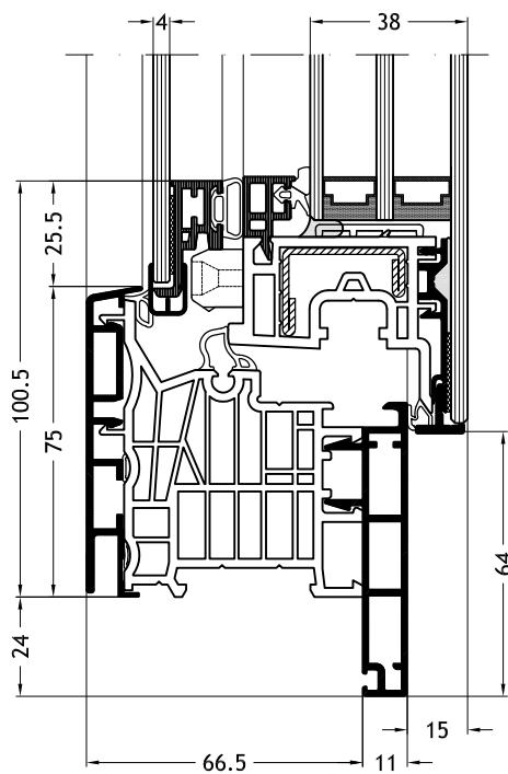
Aro em forma de L D1W com folha Nova-line Cristal Twin A34
