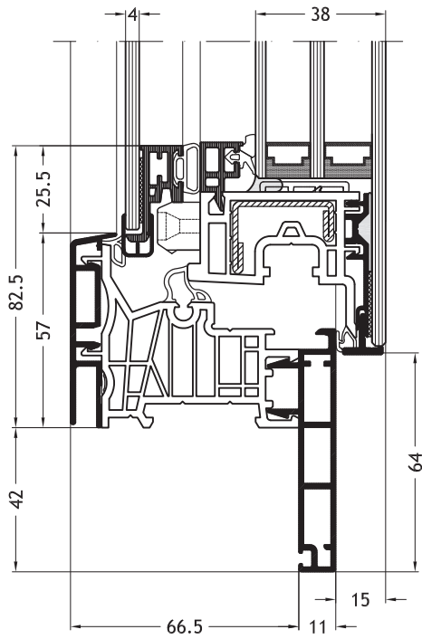
Aro em forma de Z D2V com folha Nova-line Cristal Twin A34
