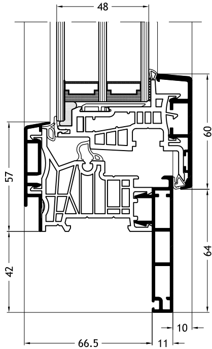
Blendrahmen Z-Form D2Y mit Flügel Nova-line Plus A24
