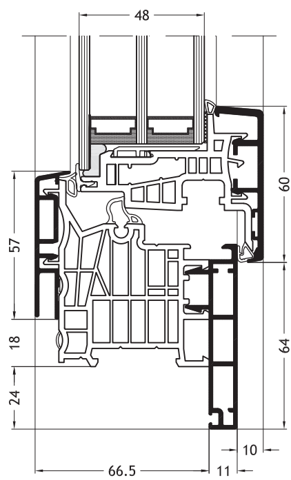
Blendrahmen L-Form D1V mit Flügel Nova-line Plus A24
