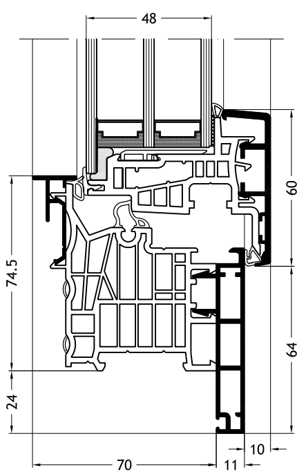
Blendrahmen L-Form D1X mit Flügel Nova-line Plus A24
