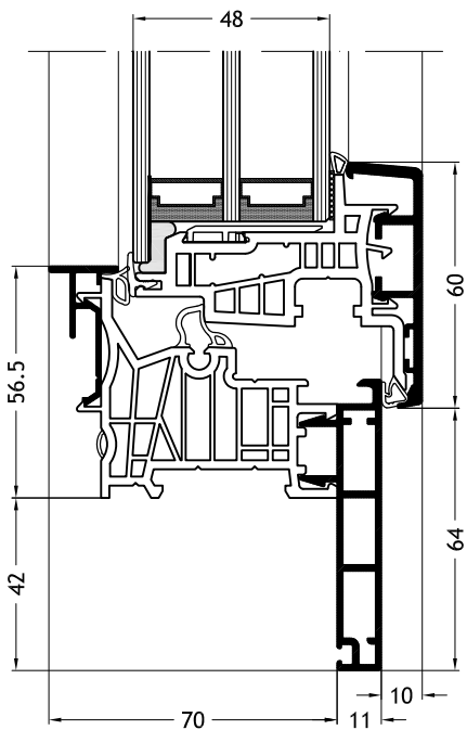
Blendrahmen Z-Form D2X mit Flügel Nova-line Plus A24
