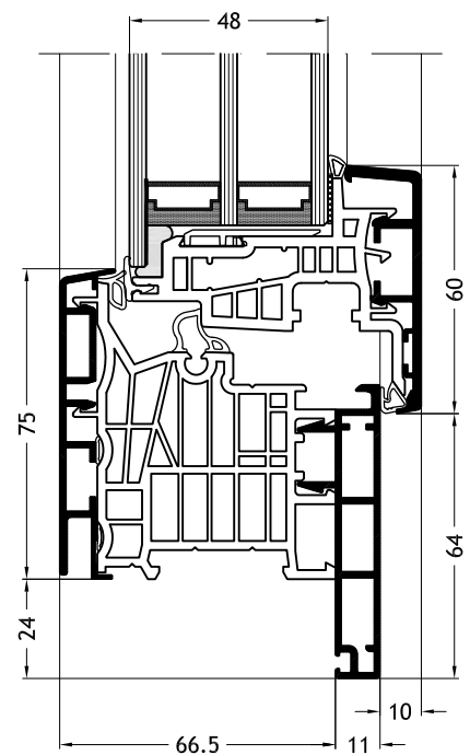
Blendrahmen L-Form D1W mit Flügel Nova-line Plus A24
