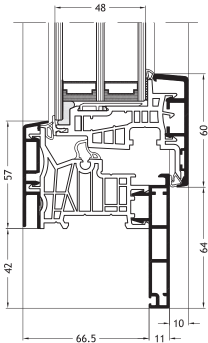
Blendrahmen Z-Form D2V mit Flügel Nova-line Plus A24
