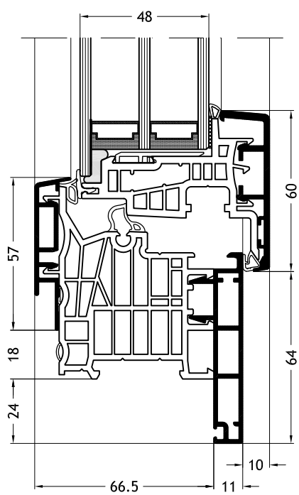
Blendrahmen L-Form D1Y mit Flügel Nova-line Plus A24
