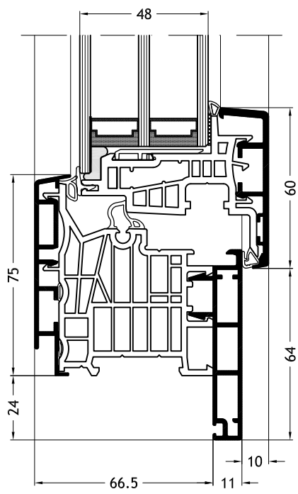
Blendrahmen L-Form D1Z mit Flügel Nova-line Plus A24
