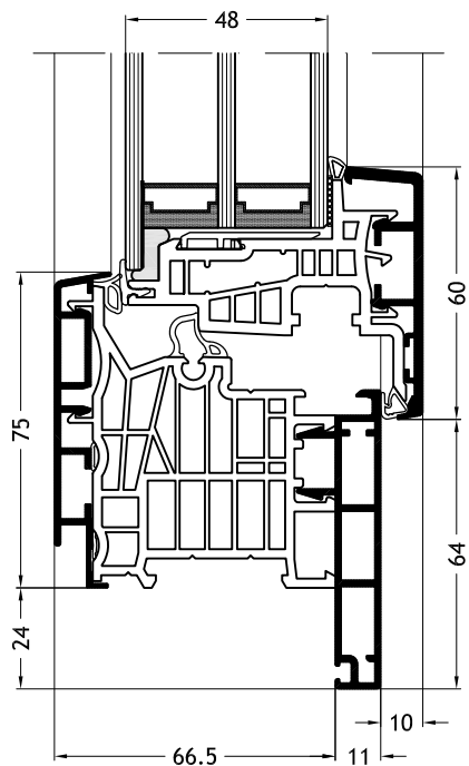
Telaio a L D1Z con anta Nova-line Plus A24
