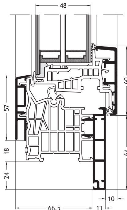
Telaio a L D1V con anta Nova-line Plus A24
