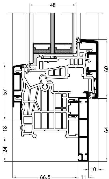
Telaio a L D1Y con anta Nova-line Plus A24
