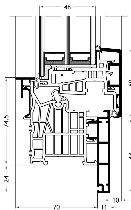
Telaio a L D1X con anta Nova-line Plus A24
