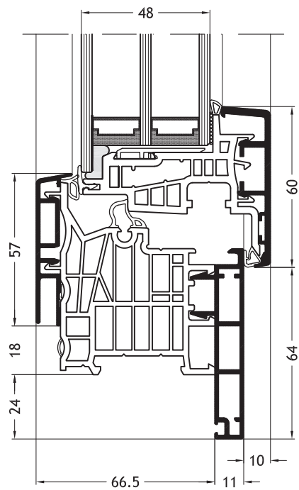
Dormant en L, D1V avec ouvrant Nova-line Plus A24
