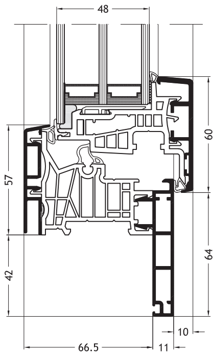
Dormant en Z, D2V avec ouvrant Nova-line Plus A24
