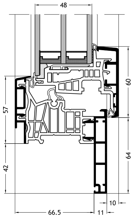
Dormant en Z, D2Y avec ouvrant Nova-line Plus A24
