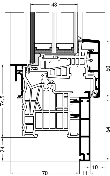
Dormant en L, D1X avec ouvrant Nova-line Plus A24
