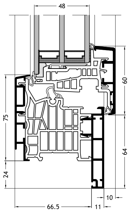
Dormant en L, D1Z avec ouvrant Nova-line Plus A24
