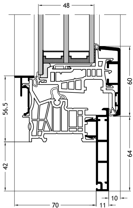
Dormant en Z, D2X avec ouvrant Nova-line Plus A24
