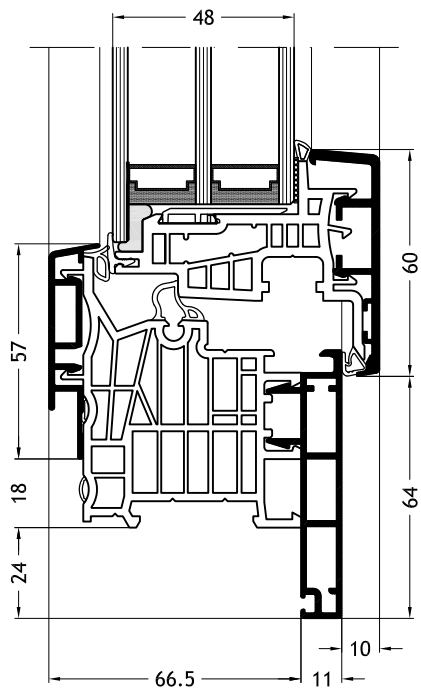
Dormant en L, D1Y avec ouvrant Nova-line Plus A24
