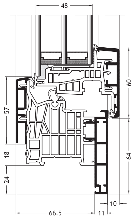
Frame L-vorm D1V met vleugel Nova-line Plus A24
