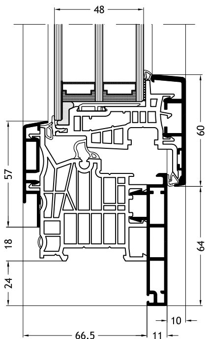
Frame L-vorm D1Y met vleugel Nova-line Plus A24
