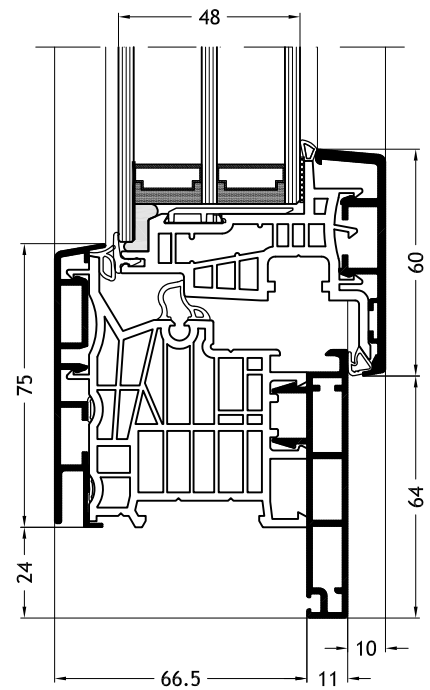
Frame L-vorm D1W met vleugel Nova-line Plus A24
