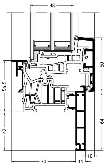
Frame Z-vorm D2X met vleugel Nova-line Plus A24
