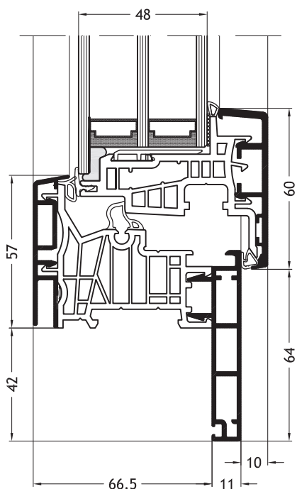
Frame Z-vorm D2V met vleugel Nova-line Plus A24
