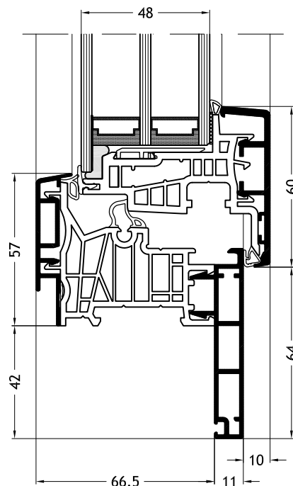
Frame Z-vorm D2Y met vleugel Nova-line Plus A24
