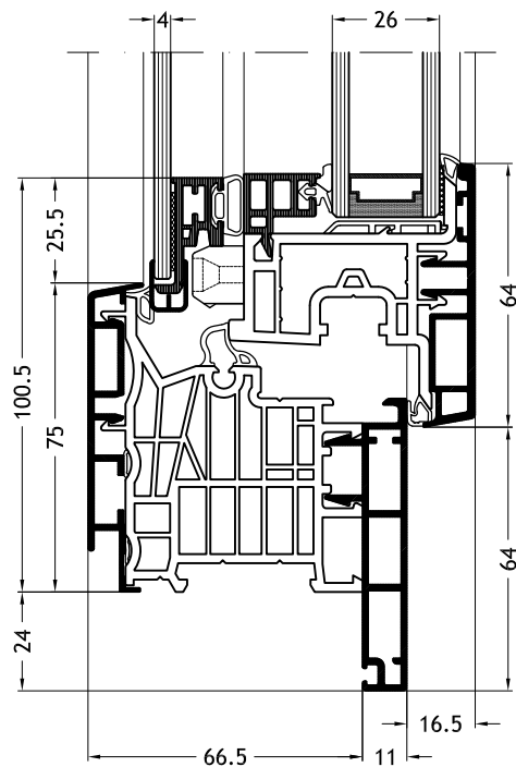
Blendrahmen L-Form D1Z mit Flügel Nova-line Twin A32
