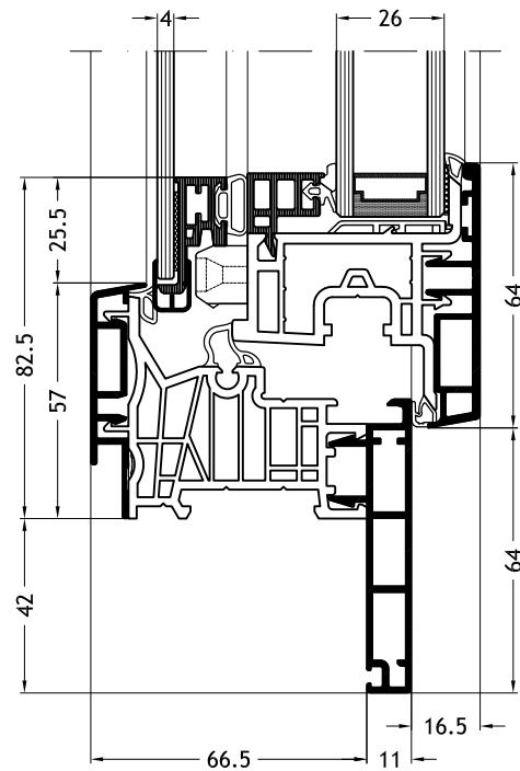
Blendrahmen Z-Form D2Y mit Flügel Nova-line Twin A32
