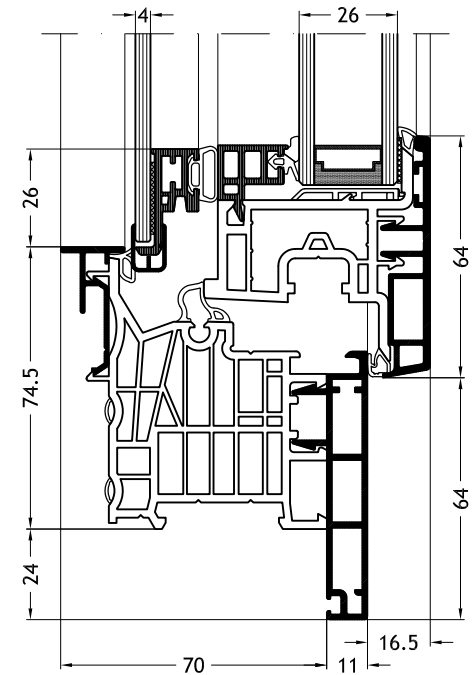
Blendrahmen L-Form D1X mit Flügel Nova-line Twin A32
