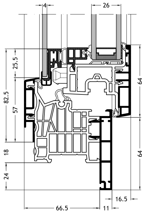
Blendrahmen L-Form D1Y mit Flügel Nova-line Twin A32
