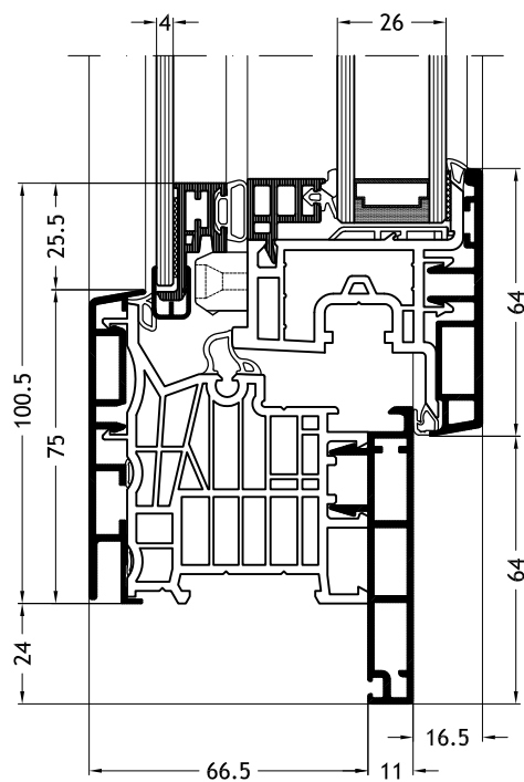
Blendrahmen L-Form D1W mit Flügel Nova-line Twin A32
