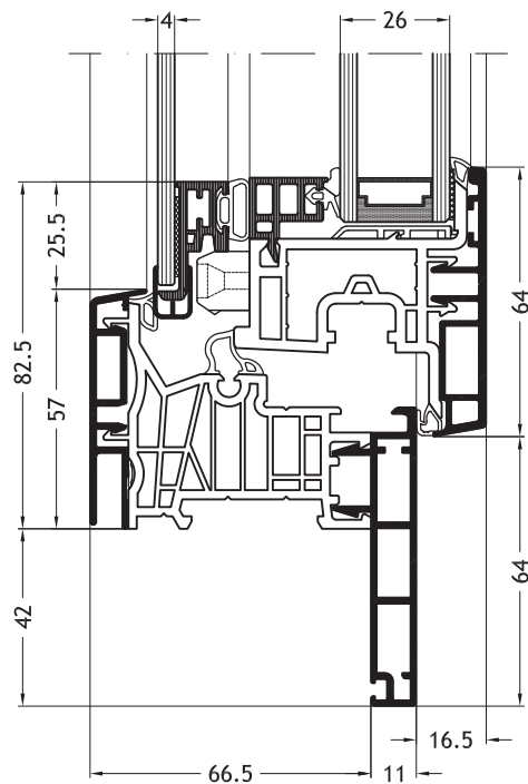
Blendrahmen Z-Form D2V mit Flügel Nova-line Twin A32
