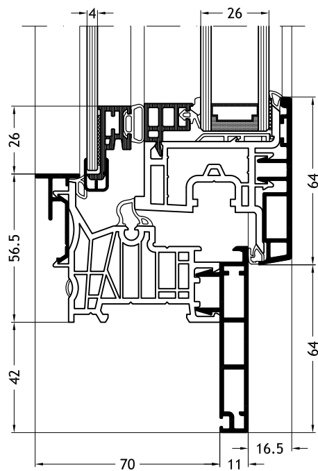
Blendrahmen Z-Form D2X mit Flügel Nova-line Twin A32
