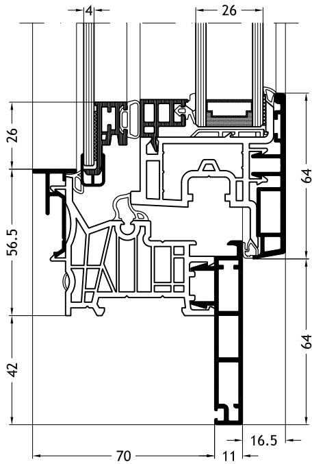
Telaio a Z D2X con anta Nova-line Twin A32
