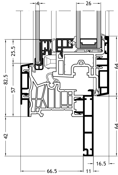
Telaio a Z D2Y con anta Nova-line Twin A32
