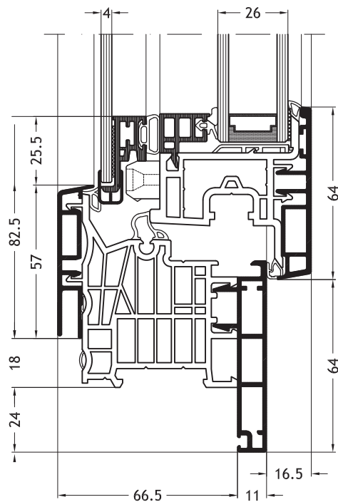
Telaio a L D1V con anta Nova-line Twin A32
