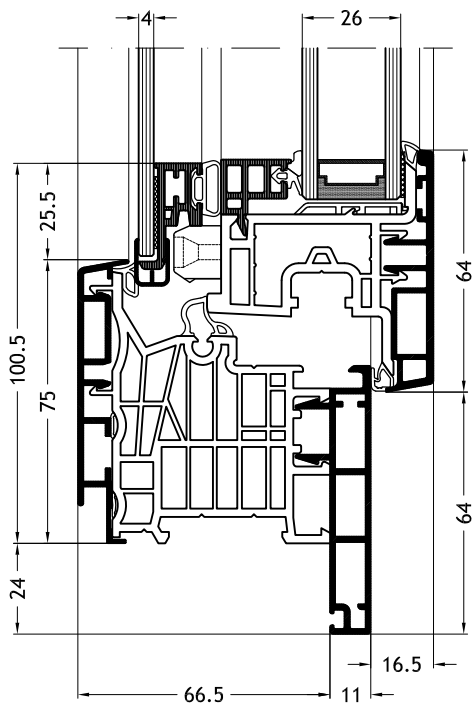
Telaio a L D1Z con anta Nova-line Twin A32
