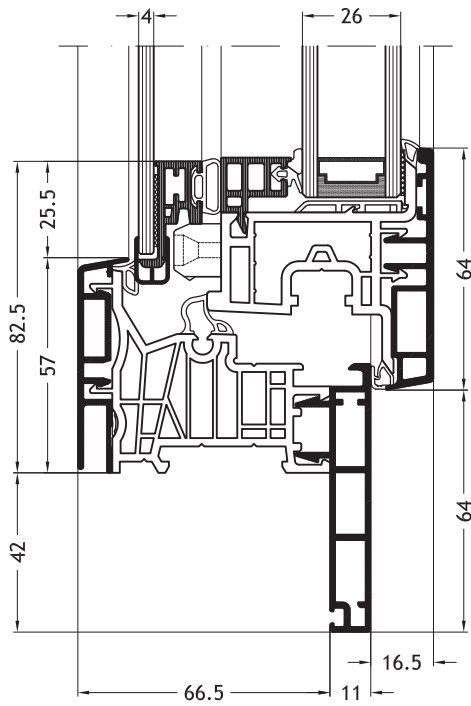
Telaio a Z D2V con anta Nova-line Twin A32
