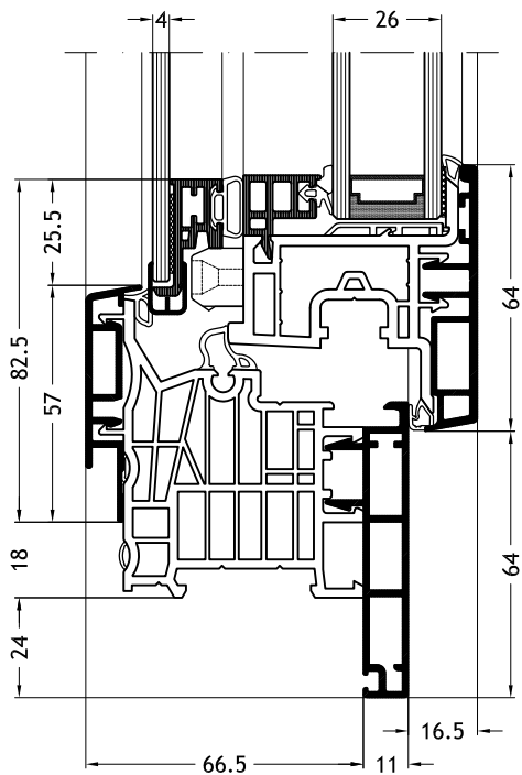
Telaio a L D1Y con anta Nova-line Twin A32
