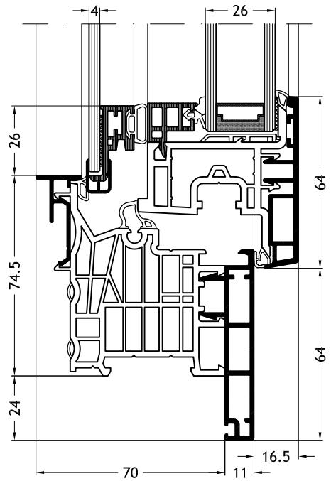
Telaio a L D1X con anta Nova-line Twin A32
