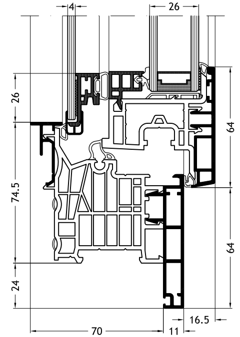
Dormant en L, D1X avec ouvrant Nova-line Twin A32
