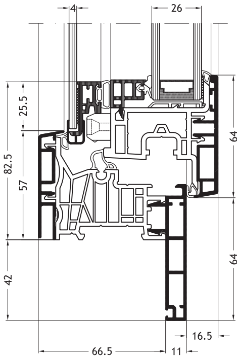
Dormant en Z, D2V avec ouvrant Nova-line Twin A32
