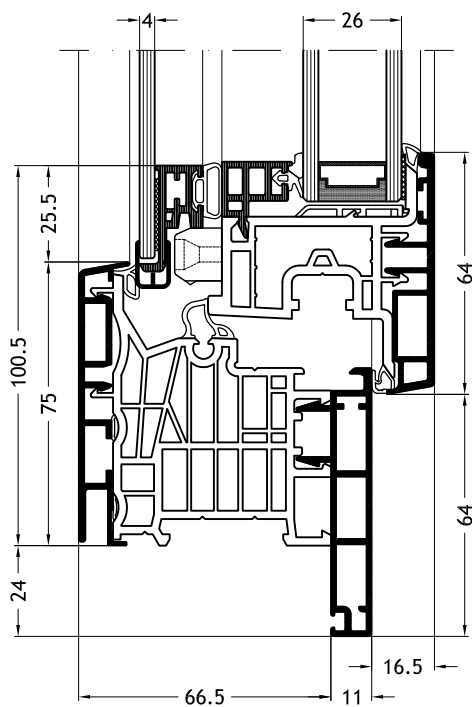
Dormant en L, D1W avec ouvrant Nova-line Twin A32
