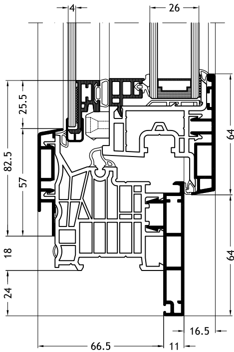
Dormant en L, D1Y avec ouvrant Nova-line Twin A32
