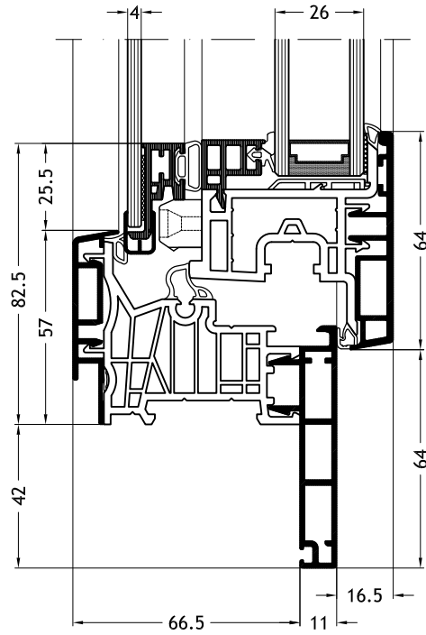
Dormant en Z, D2Y avec ouvrant Nova-line Twin A32
