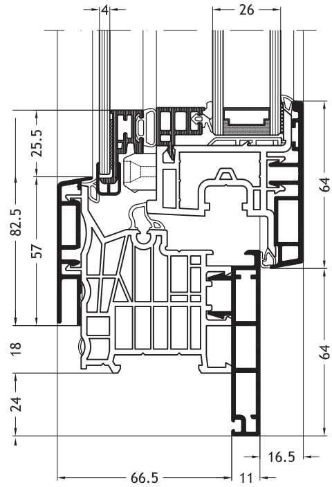
Dormant en L, D1V avec ouvrant Nova-line Twin A32
