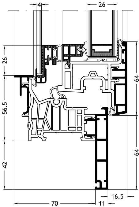
Dormant en Z, D2X avec ouvrant Nova-line Twin A32
