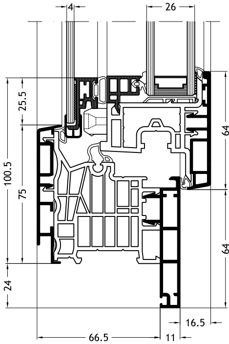
Dormant en L, D1Z avec ouvrant Nova-line Twin A32
