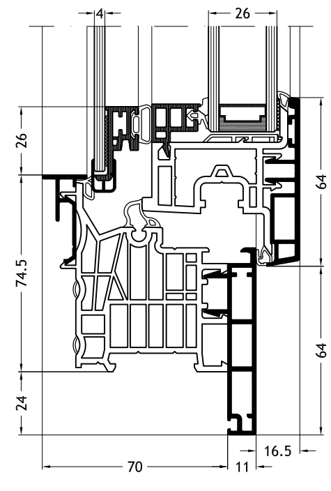
Frame L-vorm D1X met vleugel Nova-line Twin A32
