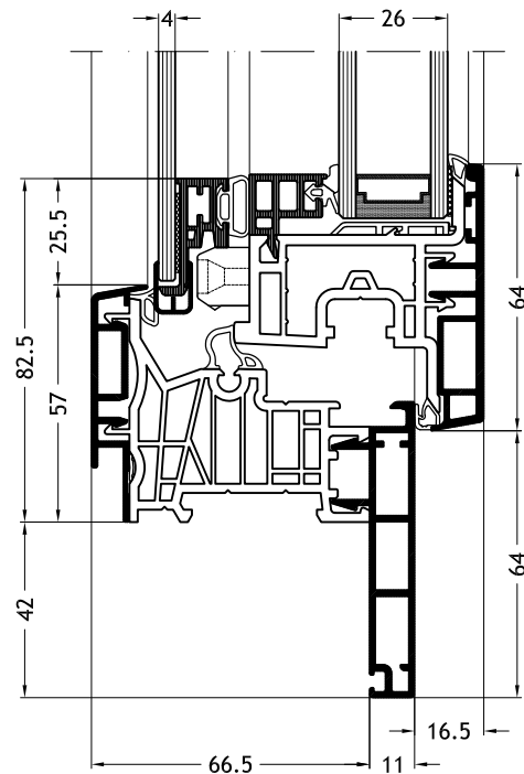
Frame Z-vorm D2Y met vleugel Nova-line Twin A32
