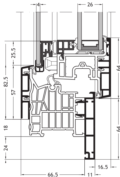
Frame L-vorm D1V met vleugel Nova-line Twin A32
