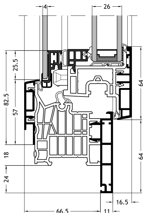
Frame L-vorm D1Y met vleugel Nova-line Twin A32
