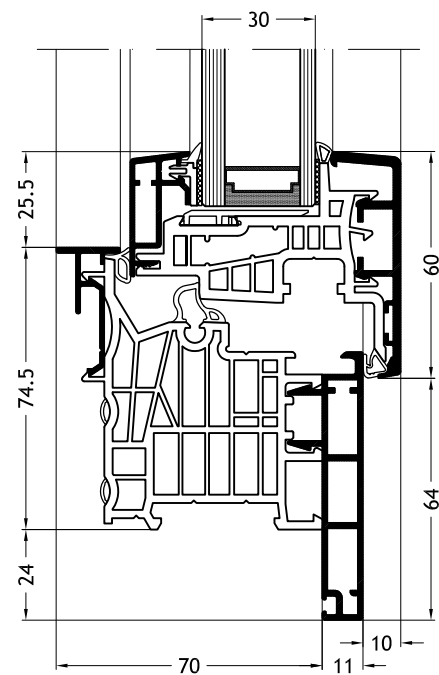
Blendrahmen L-Form D1X mit Flügel Step-line A25
