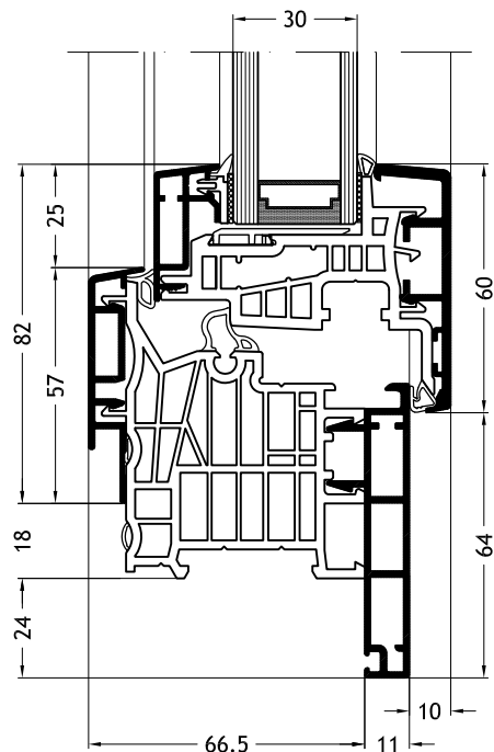
Blendrahmen L-Form D1Y mit Flügel Step-line A25
