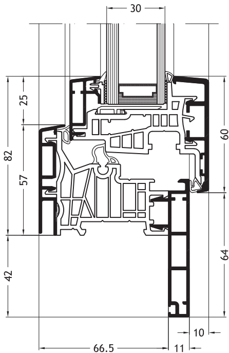
Blendrahmen Z-Form D2V mit Flügel Step-line A25
