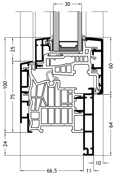
Blendrahmen L-Form D1Z mit Flügel Step-line A25
