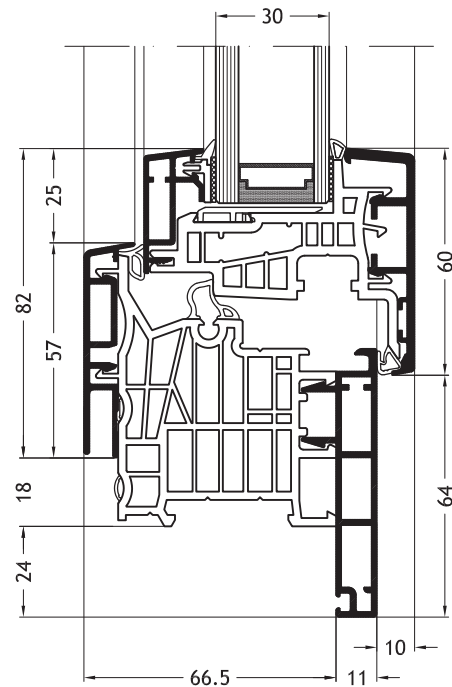
Blendrahmen L-Form D1V mit Flügel Step-line A25
