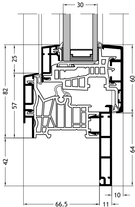
Blendrahmen Z-Form D2Y mit Flügel Step-line A25
