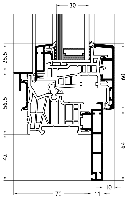
Blendrahmen Z-Form D2X mit Flügel Step-line A25
