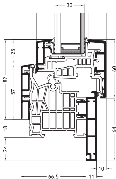
Telaio a L D1V con anta Step-line A25
