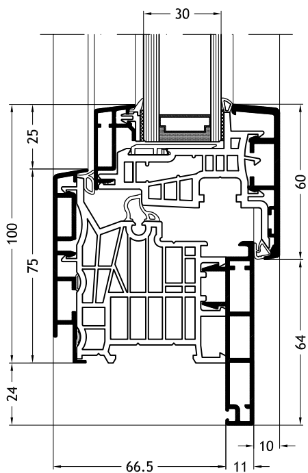
Telaio a L D1Z con anta Step-line A25
