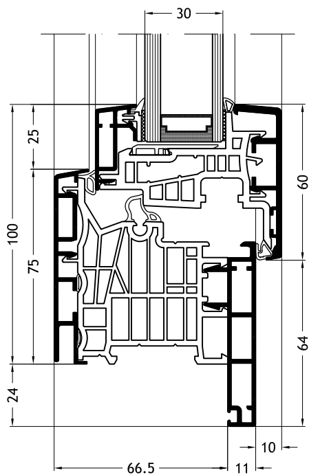
Telaio a L D1W con anta Step-line A25
