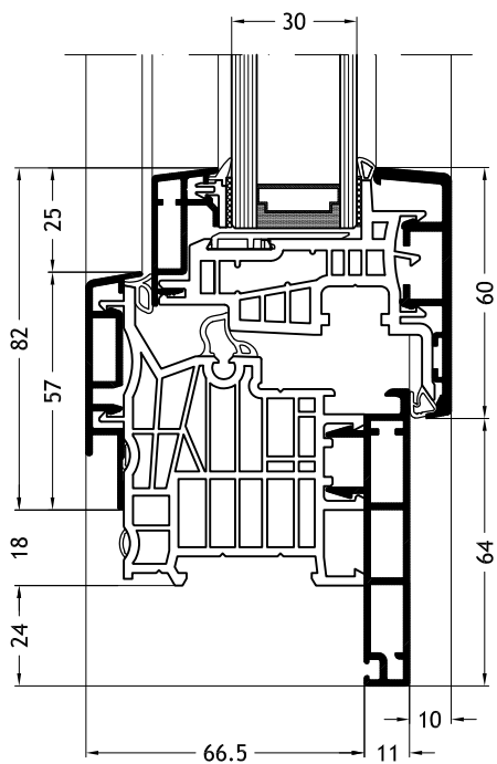
Telaio a L D1Y con anta Step-line A25
