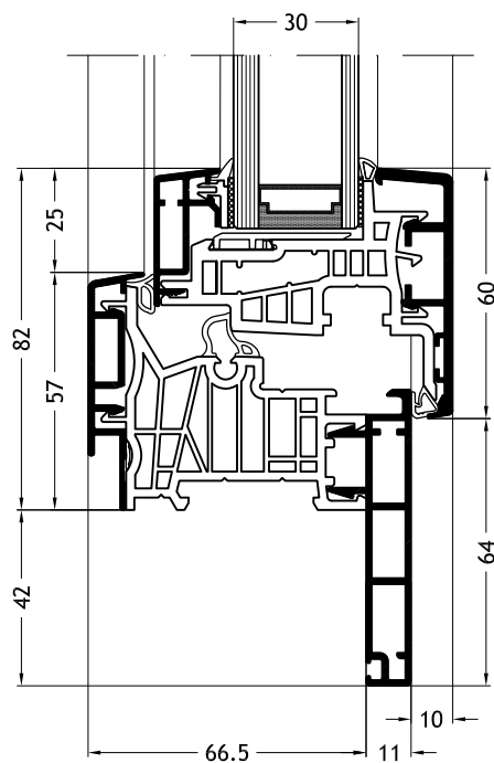
Telaio a Z D2Y con anta Step-line A25
