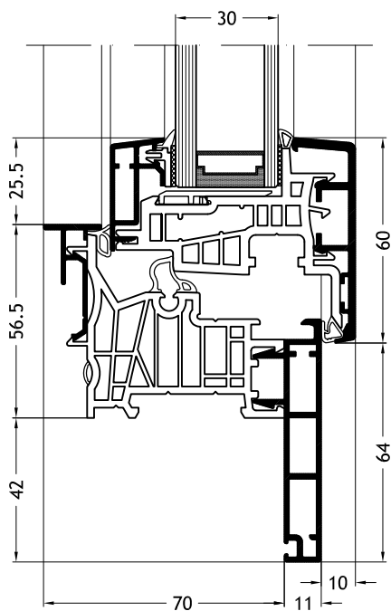
Telaio a Z D2X con anta Step-line A25
