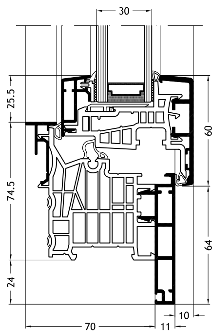
Telaio a L D1X con anta Step-line A25
