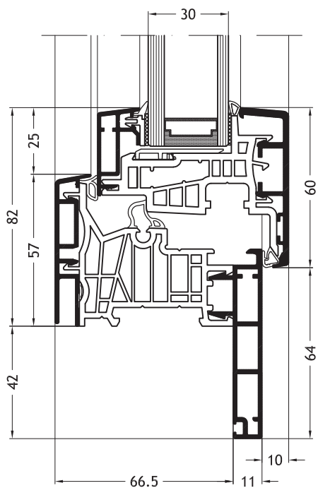
Telaio a Z D2V con anta Step-line A25
