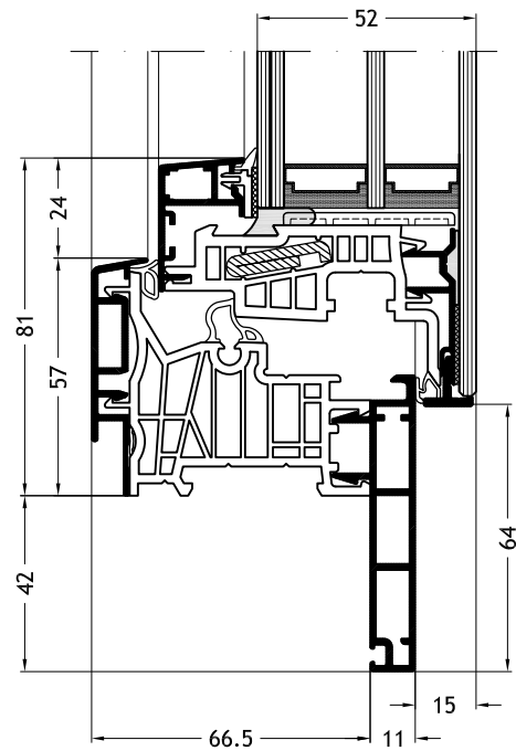
Blendrahmen Z-Form D2Y mit Flügel Step-line Cristal A23
