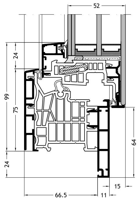
Blendrahmen L-Form D1W mit Flügel Step-line Cristal A23
