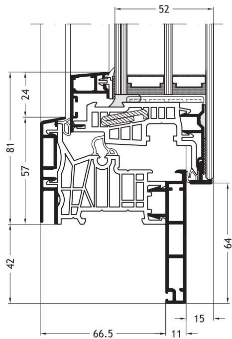
Blendrahmen Z-Form D2V mit Flügel Step-line Cristal A23
