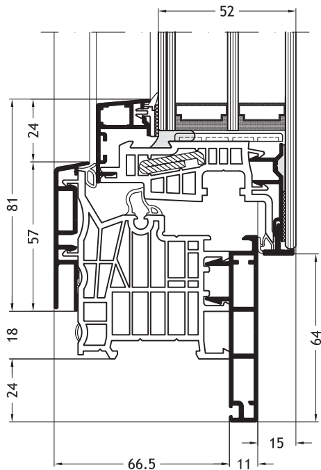
Blendrahmen L-Form D1V mit Flügel Step-line Cristal A23
