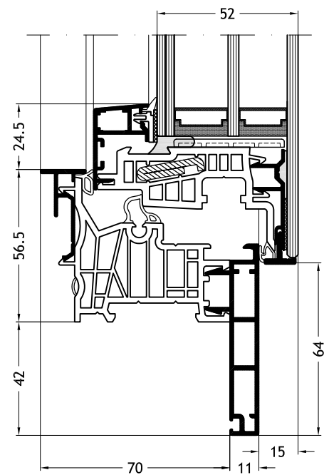
Blendrahmen Z-Form D2X mit Flügel Step-line Cristal A23
