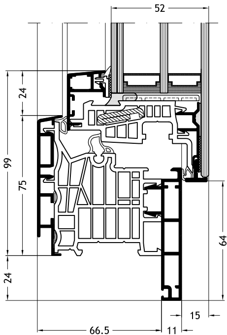
Blendrahmen L-Form D1Z mit Flügel Step-line Cristal A23
