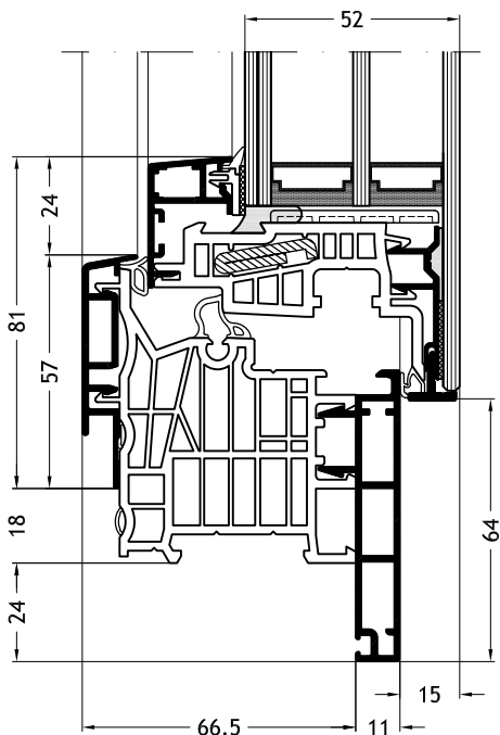
Blendrahmen L-Form D1Y mit Flügel Step-line Cristal A23
