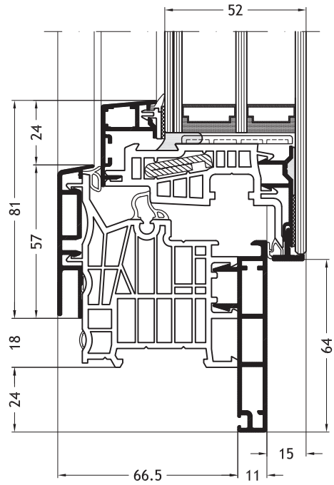
Kozijn L-vorm D1V met vleugel Step line Cristal A23
