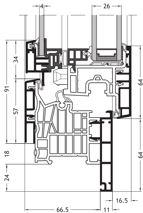
Blendrahmen L-Form D1V mit Flügel Slim-line Twin A31
