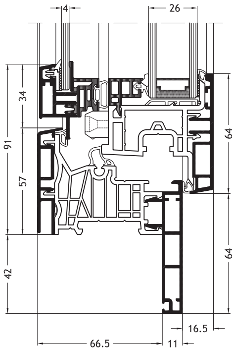
Blendrahmen Z-Form D2V mit Flügel Slim-line Twin A31
