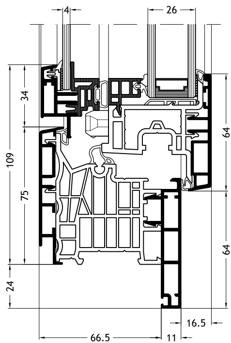
Blendrahmen L-Form D1Z mit Flügel Slim-line Twin A31
