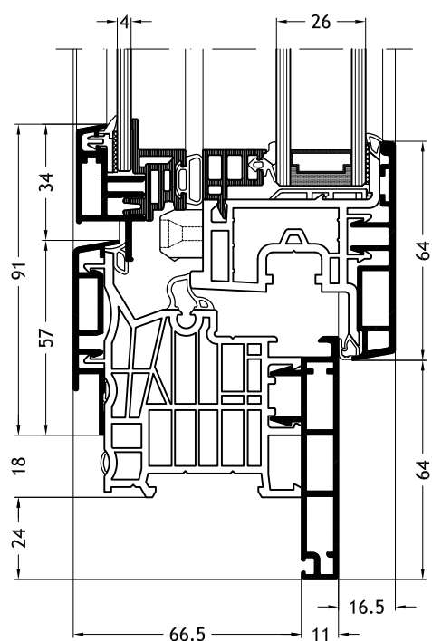
Blendrahmen L-Form D1Y mit Flügel Slim-line Twin A31
