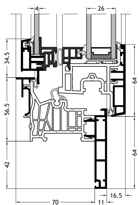
Blendrahmen Z-Form D2X mit Flügel Slim-line Twin A31
