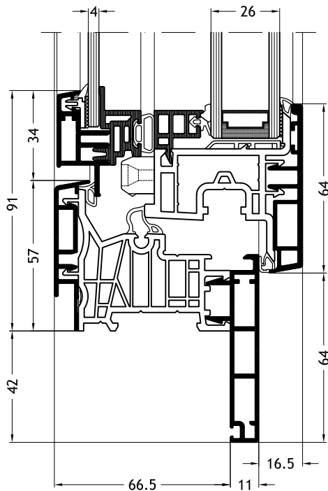
Blendrahmen Z-Form D2Y mit Flügel Slim-line Twin A31
