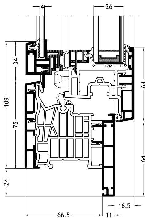
Blendrahmen L-Form D1W mit Flügel Slim-line Twin A31
