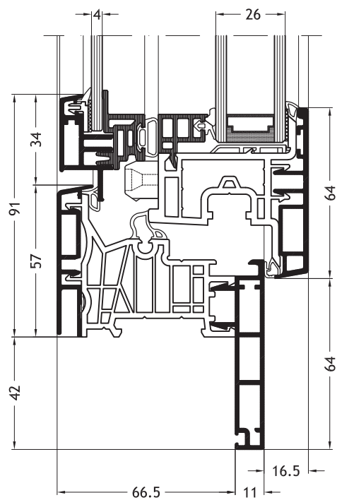
Aro em forma de Z D2V com folha Slim-line Twin A31
