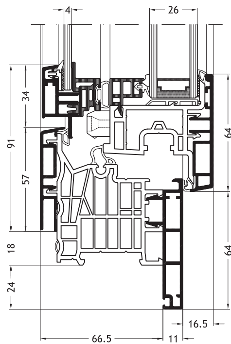
Aro em forma de L D1V com folha Slim-line Twin A31
