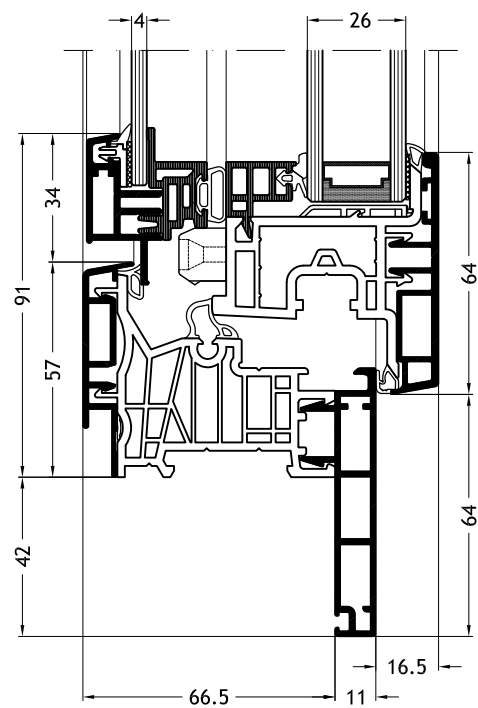
Aro em forma de Z D2Y com folha Slim-line Twin A31
