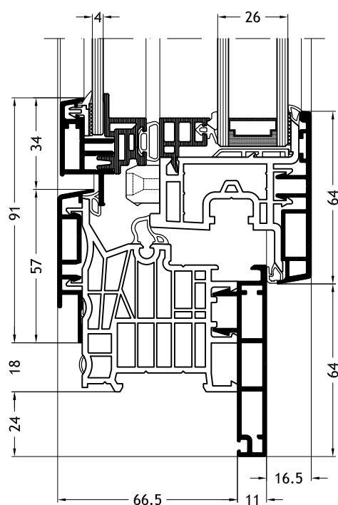
Aro em forma de L D1Y com folha Slim-line Twin A31
