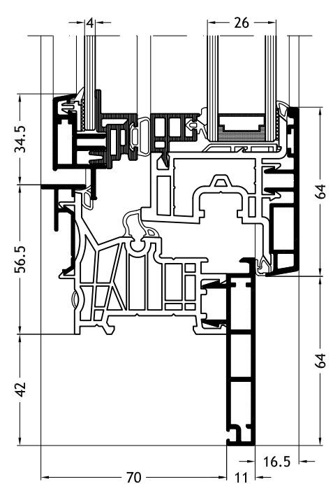
Aro em forma de Z D2X com folha Slim-line Twin A31
