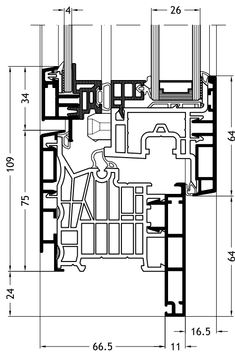
Aro em forma de L D1Z com folha Slim-line Twin A31
