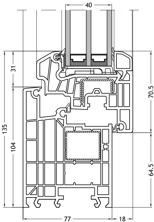
Dormant en L, 963 avec ouvrant Classic-line
