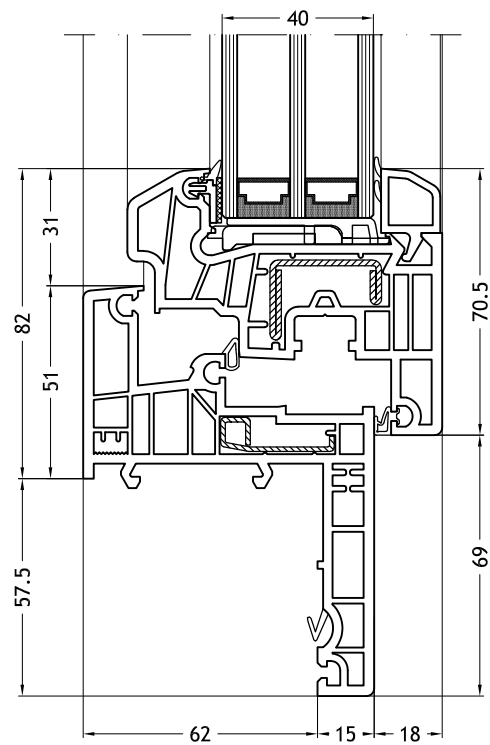
Marco Z - 966 con hoja Classic-line
