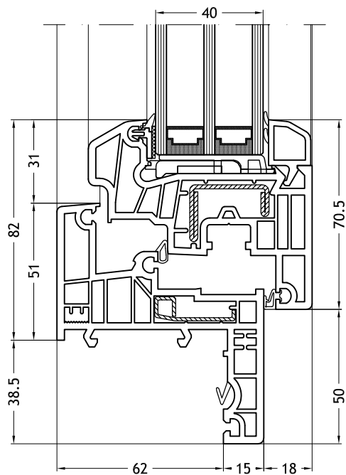
Marco Z - 965 con hoja Classic-line
