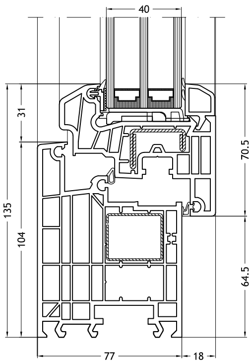
Kozijn L-vorm 963 met vleugel Classic-line
