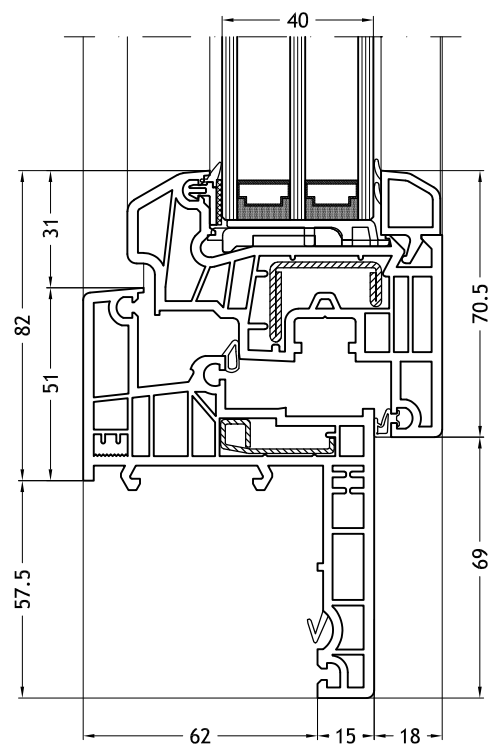
Kozijn Z-vorm 966 met vleugel Classic-line
