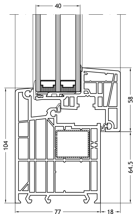
Aro em forma de Z 964 com folha Nova-line 953
