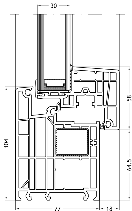
Aro em forma de Z 964 com folha Nova-line 971
