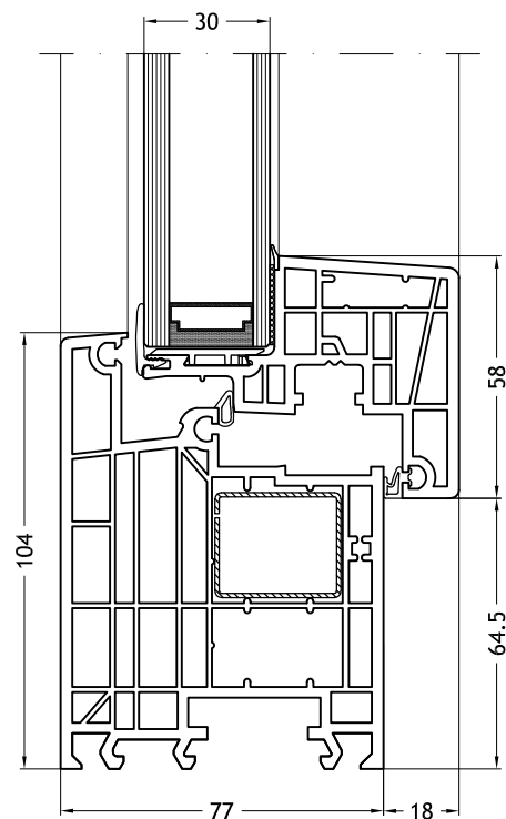
Kozijn L-vorm 963 met vleugel Nova-line 971
