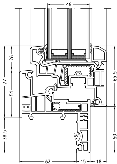
Blendrahmen Z-Form 965 mit Flügel Slim-line
