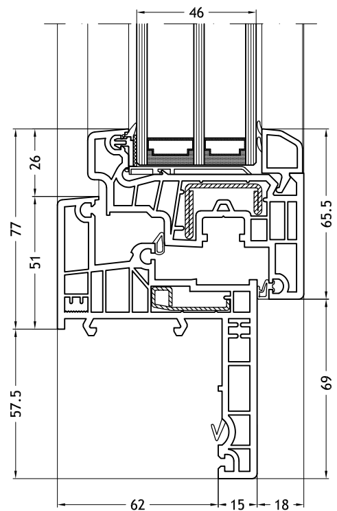
Blendrahmen Z-Form 966 mit Flügel Slim-line
