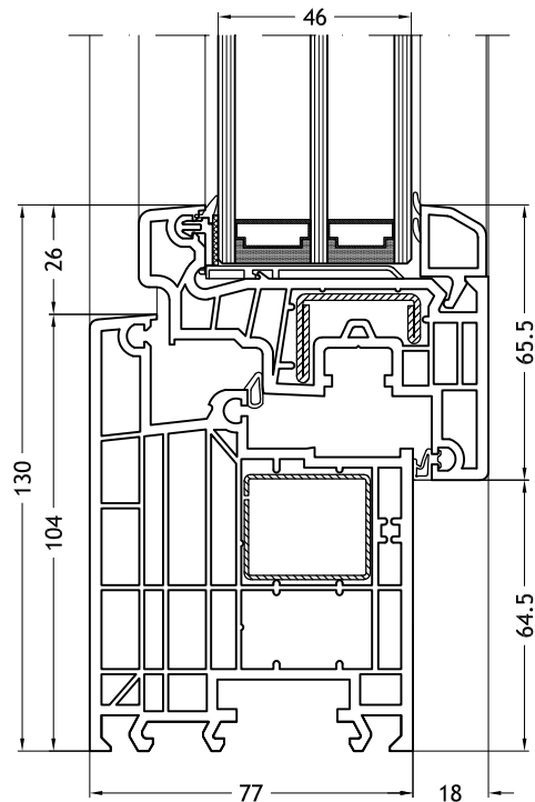
Blendrahmen L-Form 963 mit Flügel Slim-line
