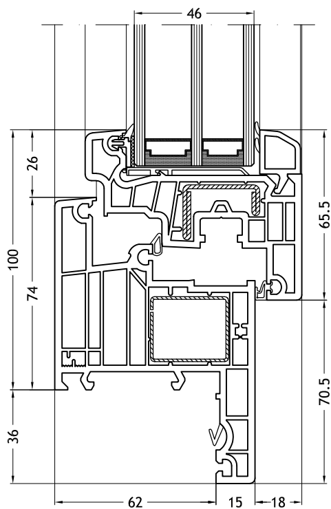
Telaio a Z 967 con anta Slim-line
