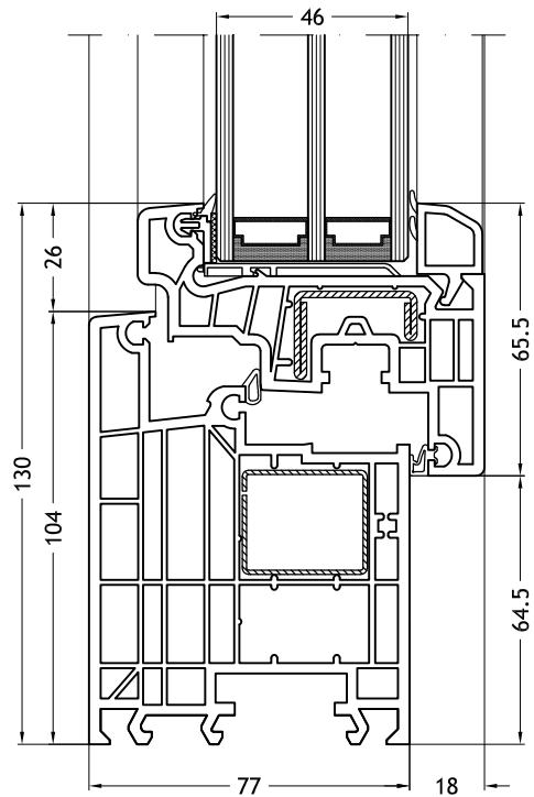
Telaio a L 963 con anta Slim-line
