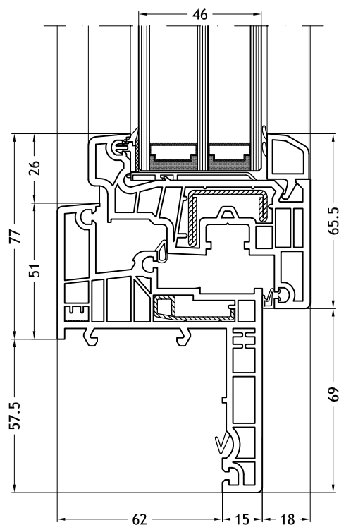
Dormant en Z, 966 avec ouvrant Slim-line
