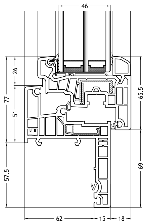
Kozijn Z-vorm 966 met vleugel Slim-line
