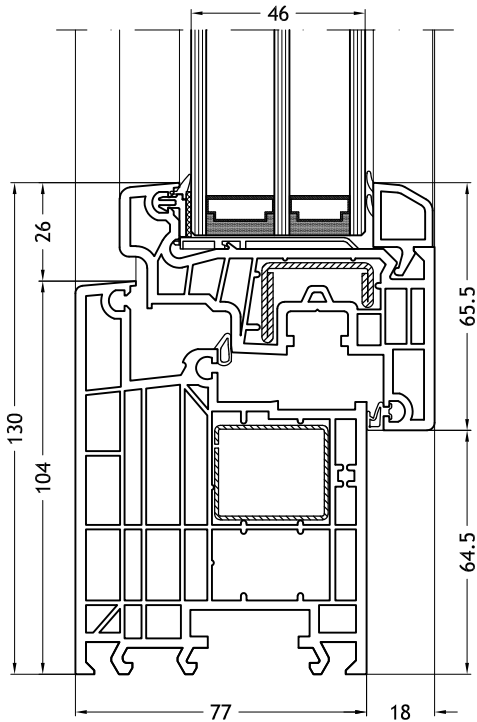
Kozijn L-vorm 963 met vleugel Slim-line
