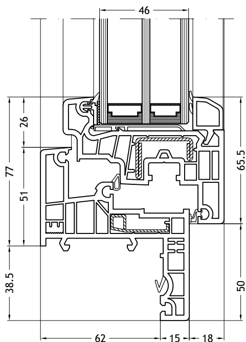
Kozijn Z-vorm 965 met vleugel Slim-line
