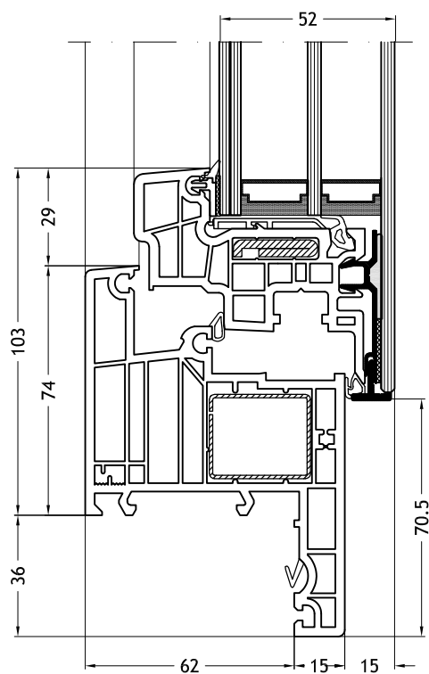
Blendrahmen Z-Form 967 mit Flügel Slim-line Cristal
