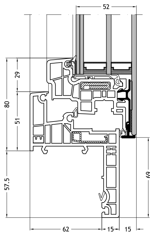
Blendrahmen Z-Form 966 mit Flügel Slim-line Cristal
