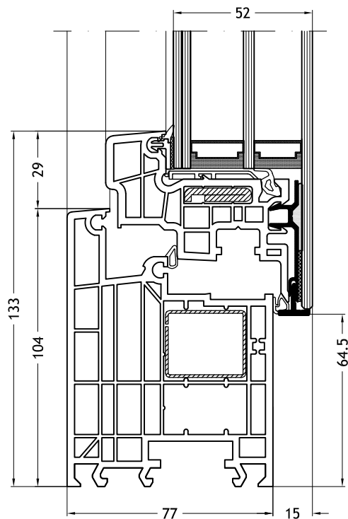
Blendrahmen L-Form 963 mit Flügel Slim-line Cristal
