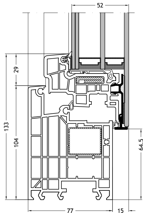
Telaio a L 963 con anta Slim-line Cristal
