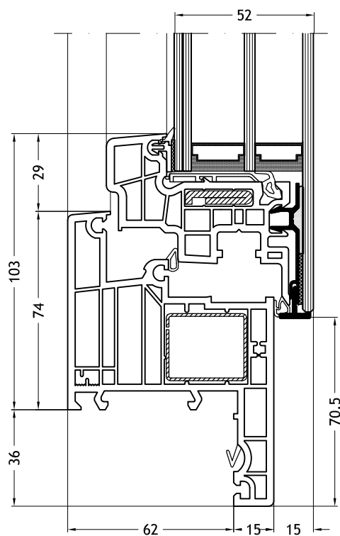
Telaio a Z 967 con anta Slim-line Cristal
