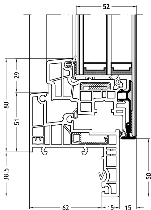
Telaio a Z 965 con anta Slim-line Cristal
