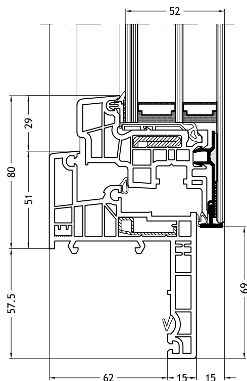
Telaio a Z 966 con anta Slim-line Cristal
