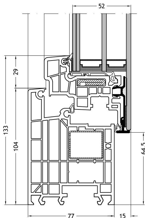
Dormant en L, 963 avec ouvrant Slim-line Cristal
