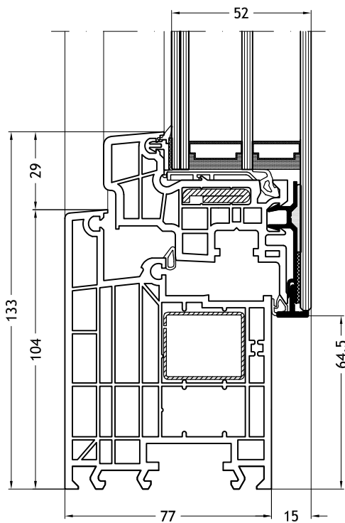
Kozijn L-vorm 963 met vleugel Slim-line Cristal
