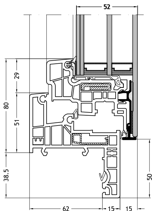
Kozijn Z-vorm 965 met vleugel Slim-line Cristal
