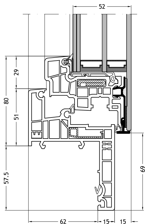
Kozijn Z-vorm 966 met vleugel Slim-line Cristal
