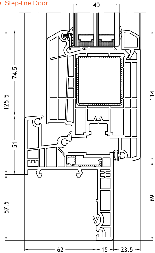
Blendrahmen Z-Form 966 mit Flügel Step-line Door
