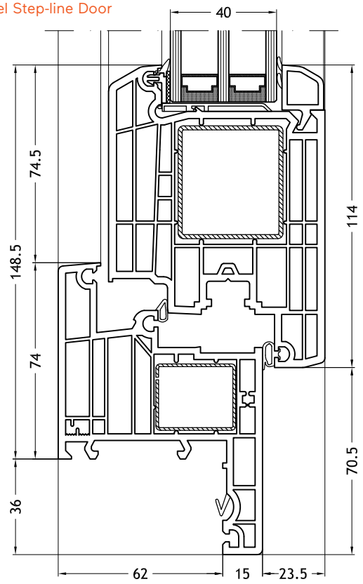
Blendrahmen Z-Form 967 mit Flügel Step-line Door
