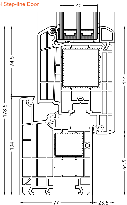
Blendrahmen L-Form 963 mit Flügel Step-line Door
