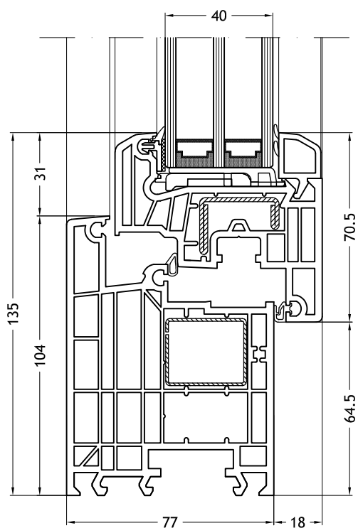
Blendrahmen L-Form 963 mit Flügel Step-line
