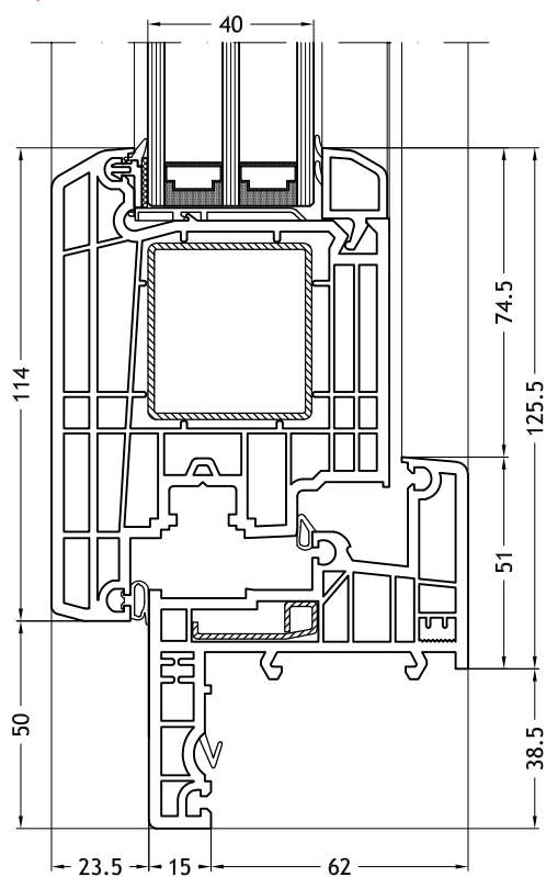
Blendrahmen Z-Form 965 mit Flügel Step-line Door out
