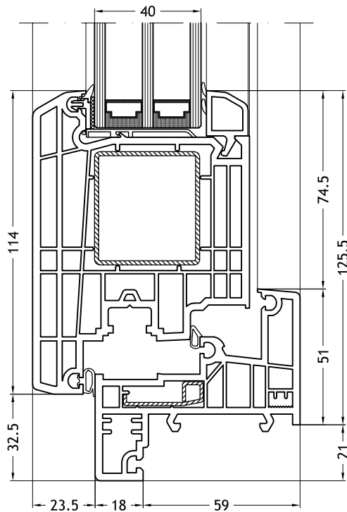
Blendrahmen Z-Form 964 mit Flügel Step-line Door out
