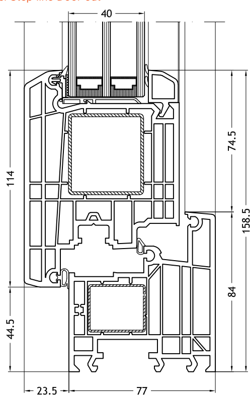
Blendrahmen L-Form 962 mit Flügel Step-line Door out
