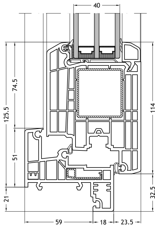
Blendrahmen Z-Form 964 mit Flügel Step-line Door
