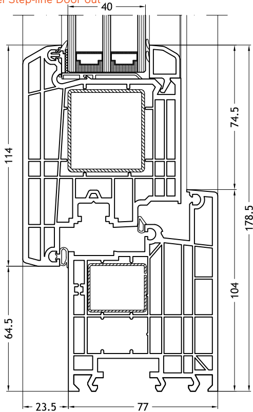
Blendrahmen L-Form 963 mit Flügel Step-line Door out
