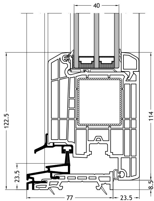
Flache Schwelle mit Flügel Step-line Door
