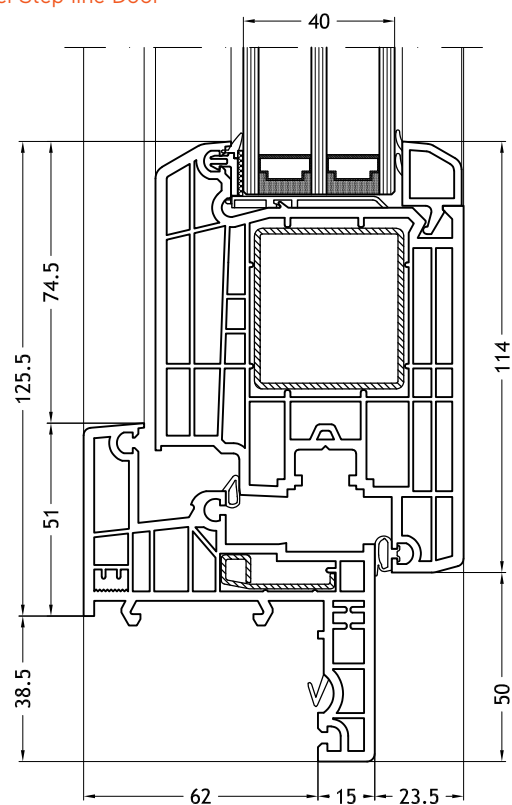
Blendrahmen Z-Form 965 mit Flügel Step-line Door
