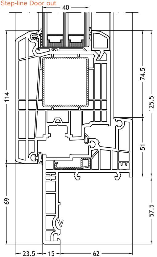
Blendrahmen Z-Form 966 mit Flügel Step-line Door out
