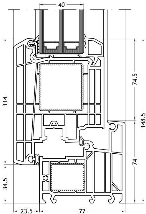
Blendrahmen L-Form 961 mit Flügel Step-line Door out
