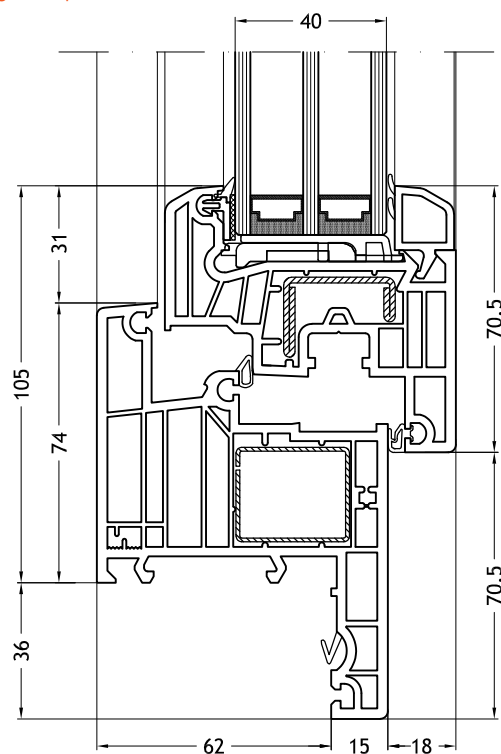
Blendrahmen Z-Form 967 mit Flügel Step-line
