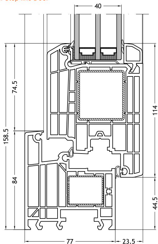
Blendrahmen L-Form 962 mit Flügel Step-line Door
