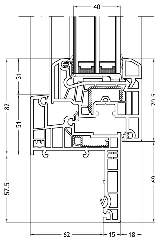
Blendrahmen Z-Form 966 mit Flügel Step-line
