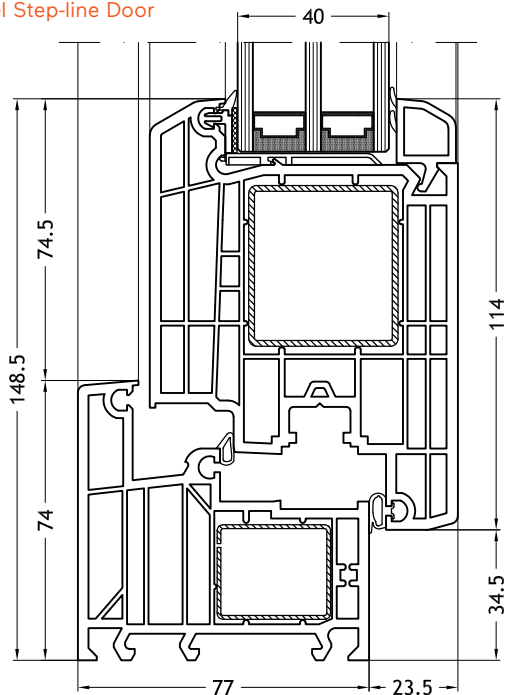
Blendrahmen L-Form 961 mit Flügel Step-line Door
