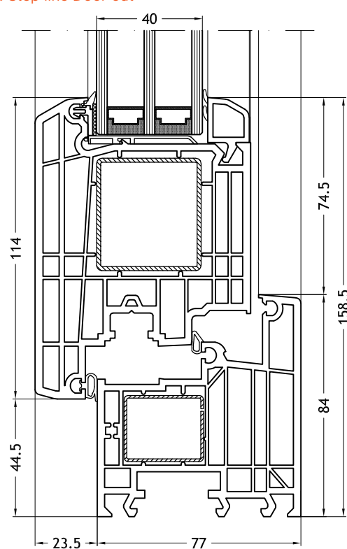
Telaio a L 962 con anta Step-line Door out
