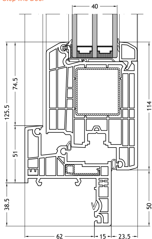
Telaio a Z 965 con anta Step-line Door
