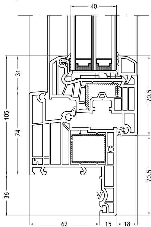
Telaio a Z 967 con anta Step-line
