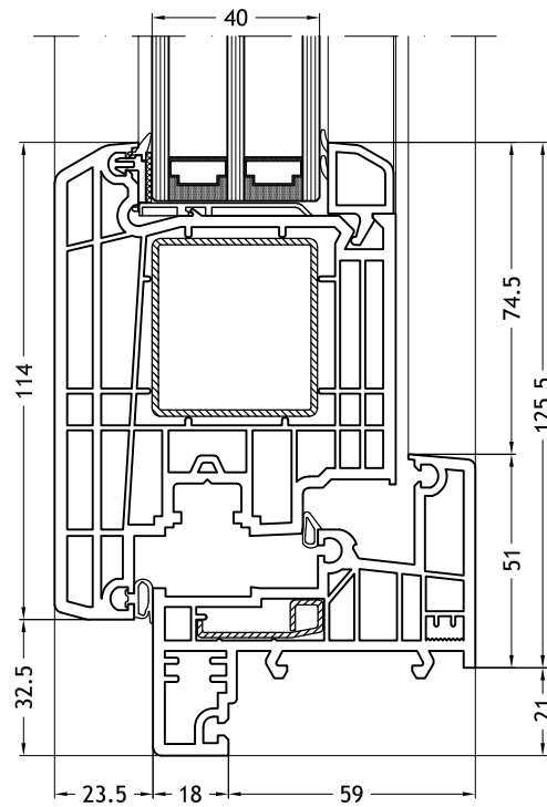
Telaio a Z 964 con anta Step-line Door out
