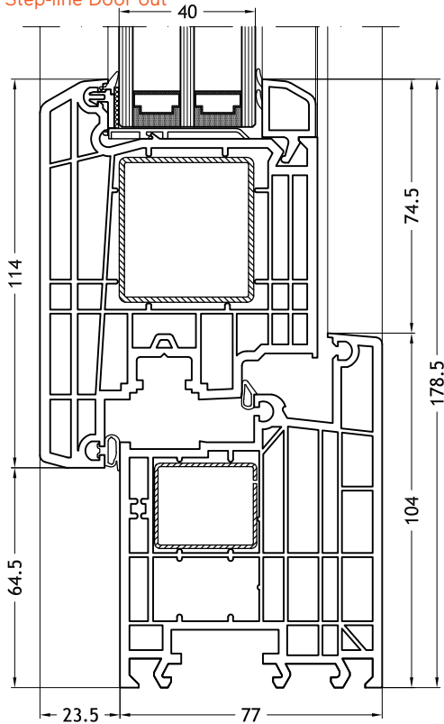
Telaio a L 963 con anta Step-line Door out
