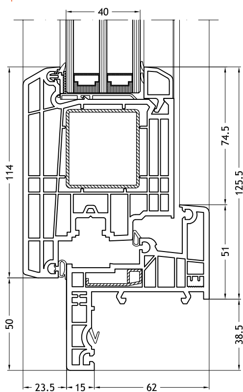
Telaio a Z 965 con anta Step-line Door out
