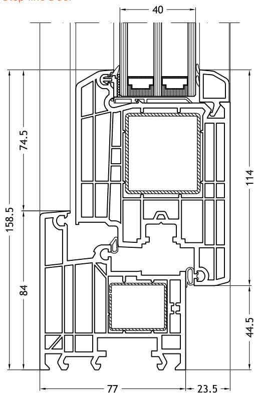
Telaio a L 962 con anta Step-line Door
