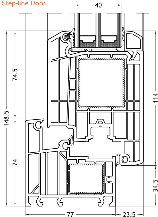
Telaio a L 961 con anta Step-line Door
