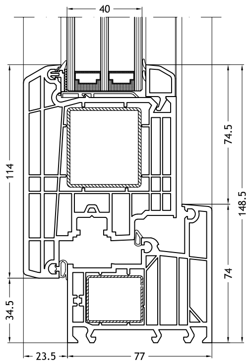
Telaio a L 961 con anta Step-line Door out
