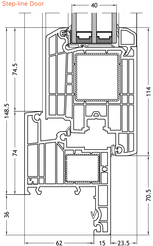
Telaio a Z 967 con anta Step-line Door
