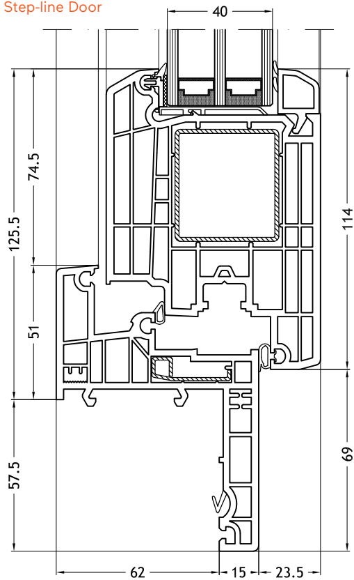
Telaio a Z 966 con anta Step-line Door
