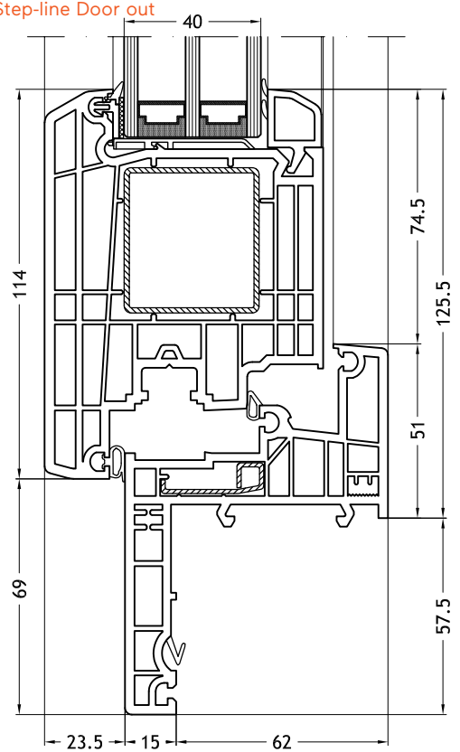
Telaio a Z 966 con anta Step-line Door out
