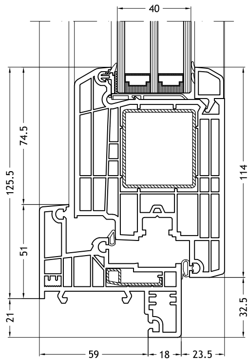
Telaio a Z 964 con anta Step-line Door
