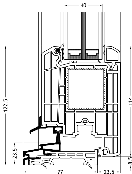
Soglia ribassata con anta Step-line Door
