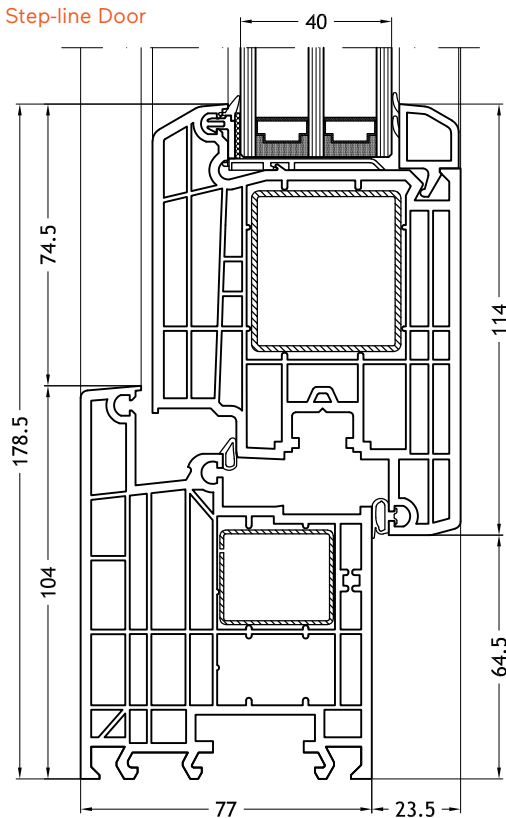
Telaio a L 963 con anta Step-line Door
