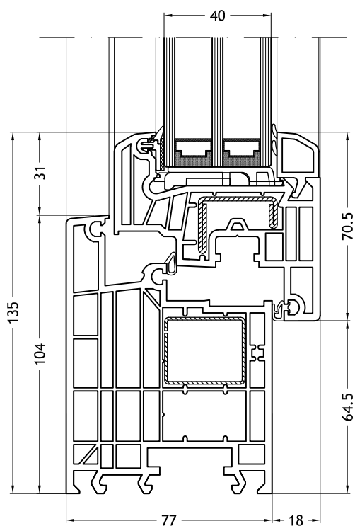
Telaio a L 963 con anta Step-line
