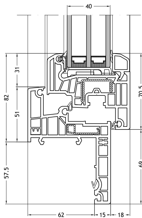
Telaio a Z 966 con anta Step-line
