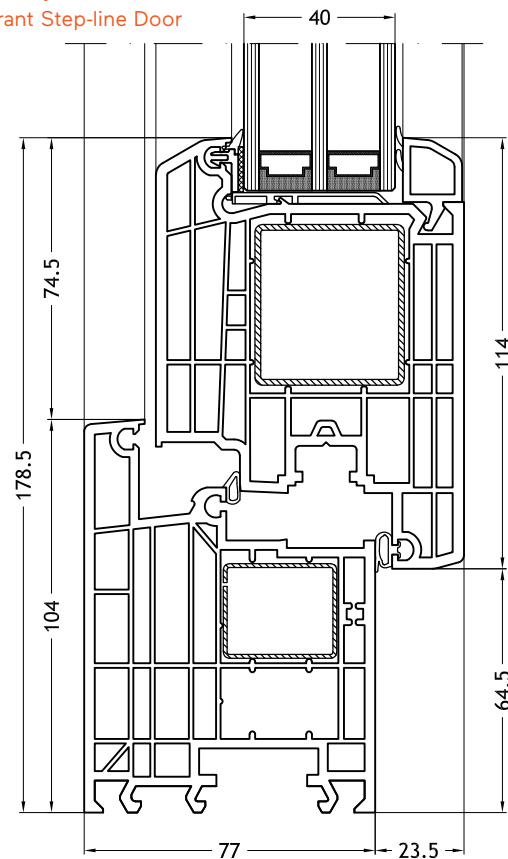
Dormant en L, 963 avec ouvrant Step-line Door
