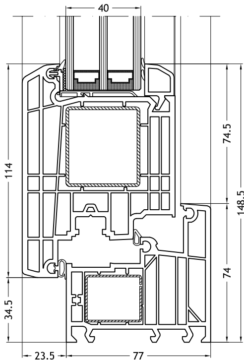
Dormant en L, 961 avec ouvrant Step-line Door out
