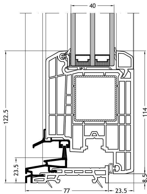
Seuil plat avec ouvrant Step-line Door
