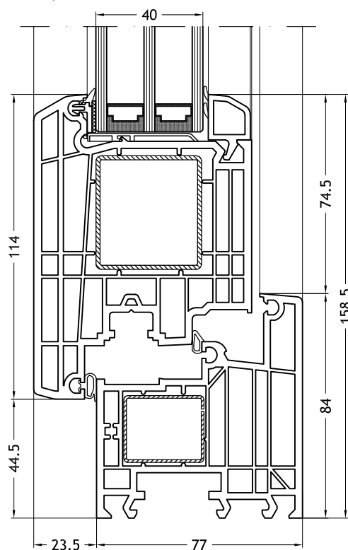
Dormant en L, 962 avec ouvrant Step-line Door out
