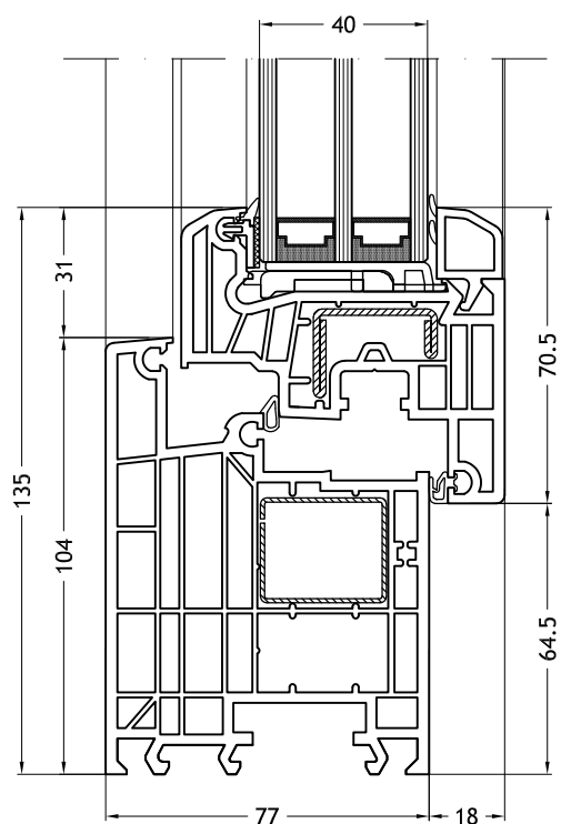
Dormant en L, 963 avec ouvrant Step-line
