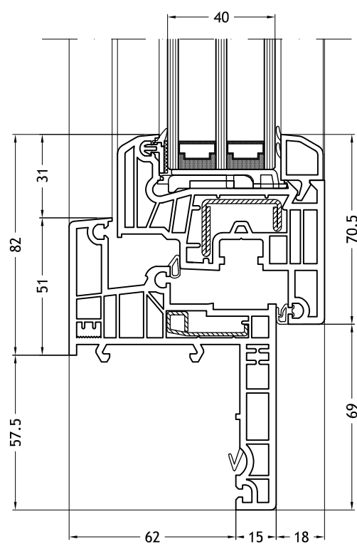
Dormant en Z, 966 avec ouvrant Step-line
