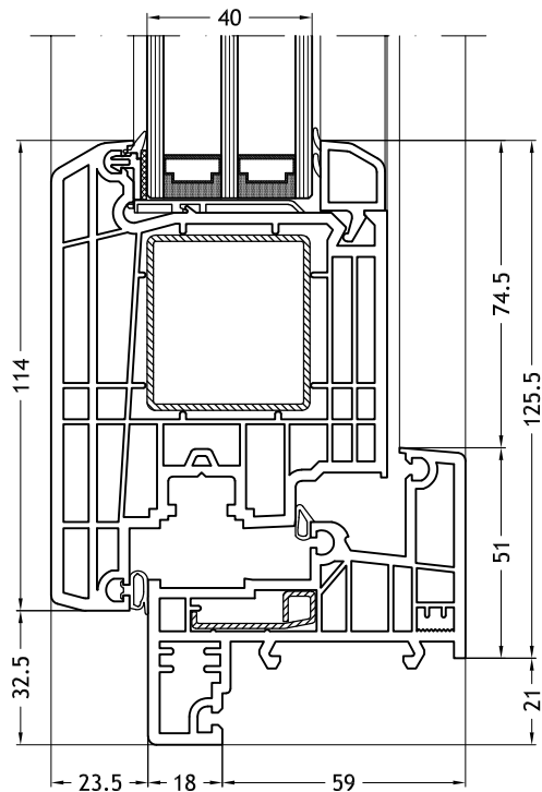
Dormant en Z, 964 avec ouvrant Step-line Door out
