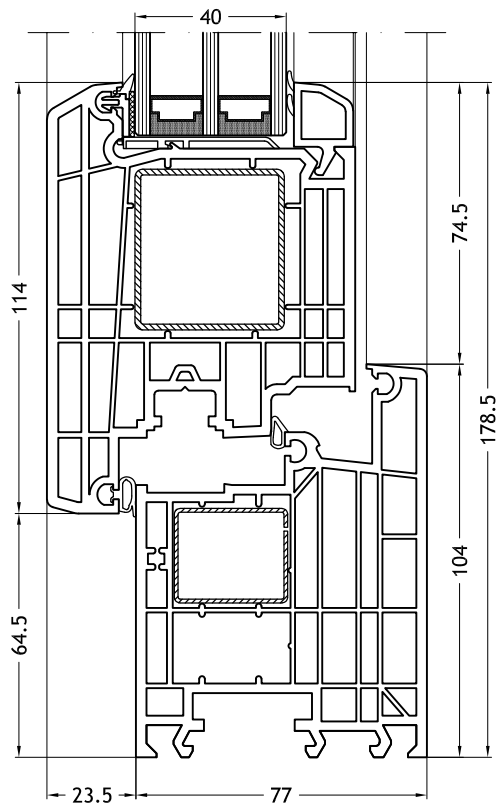
Dormant en L, 963 avec ouvrant Step-line Door out
