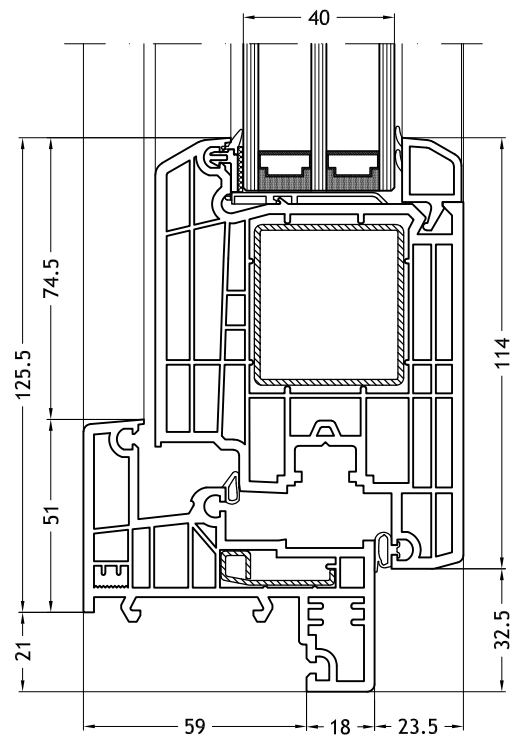
Dormant en Z, 964 avec ouvrant Step-line Door
