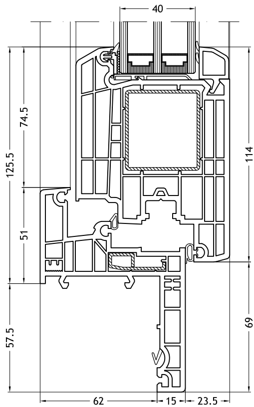
Dormant en Z, 966 avec ouvrant Step-line Door
