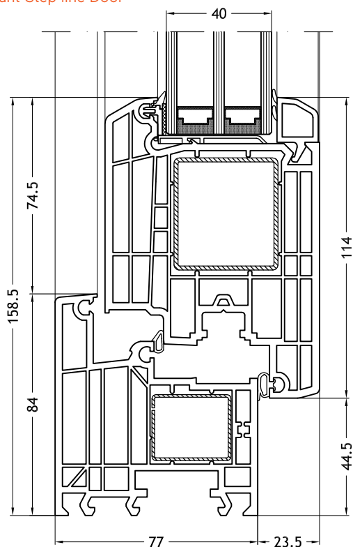
Dormant en L, 962 avec ouvrant Step-line Door
