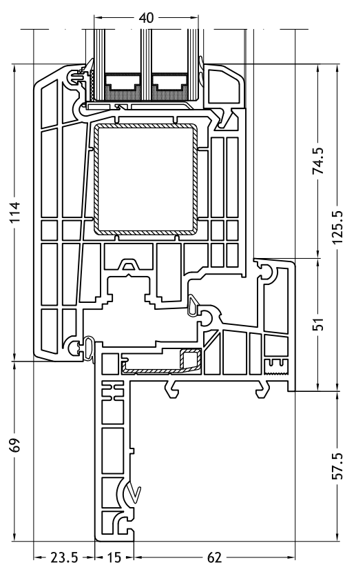
Dormant en Z, 966 avec ouvrant Step-line Door out
