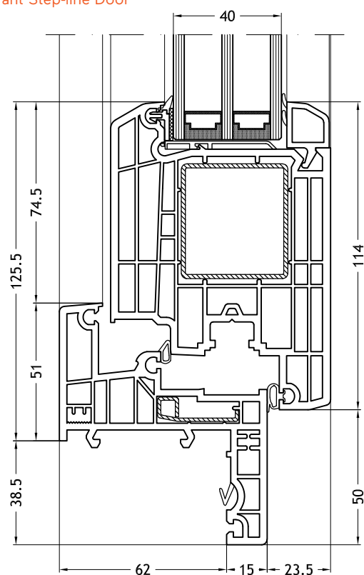
Dormant en Z, 965 avec ouvrant Step-line Door
