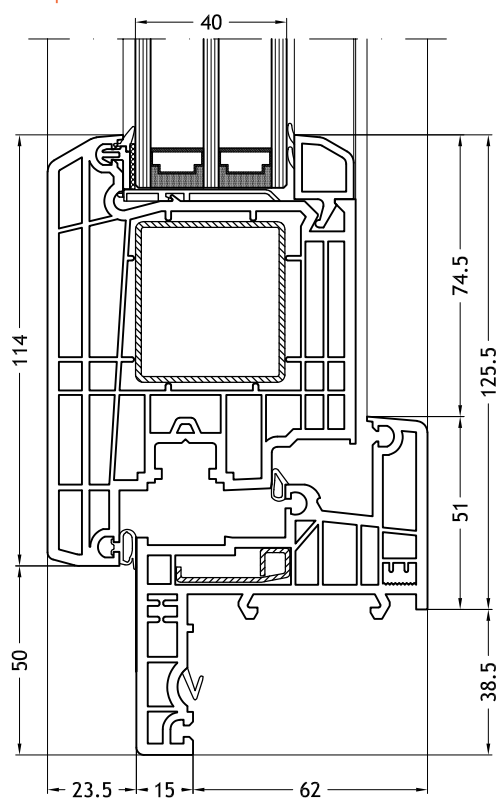
Dormant en Z, 965 avec ouvrant Step-line Door out
