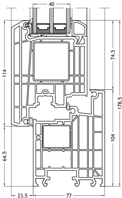
Marco L, 963 con hoja Step-line Door out
