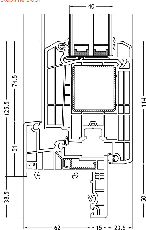
Marco Z, 965 con hoja Step-line Door
