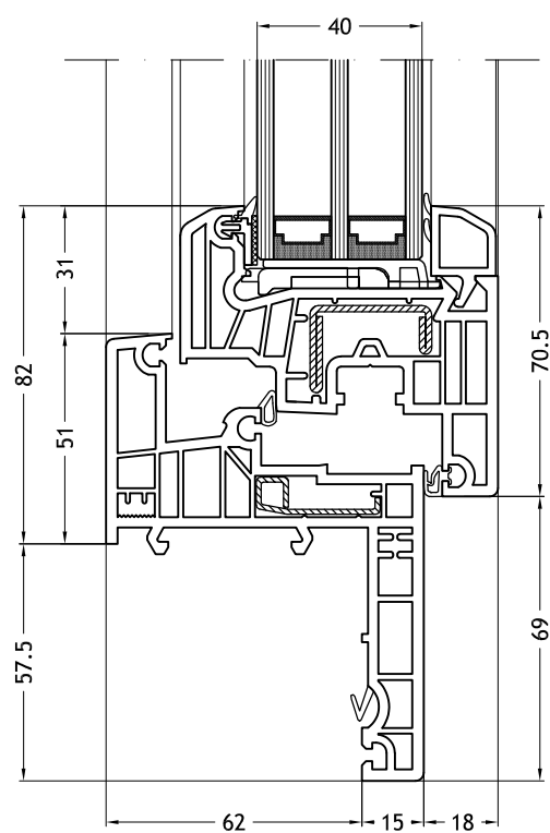
Marco Z, 966 con hoja Step-line
