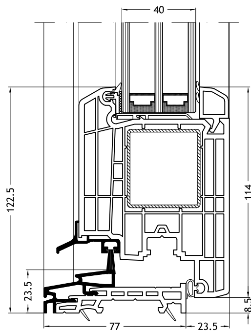
Solera plana con hoja Step-line Door
