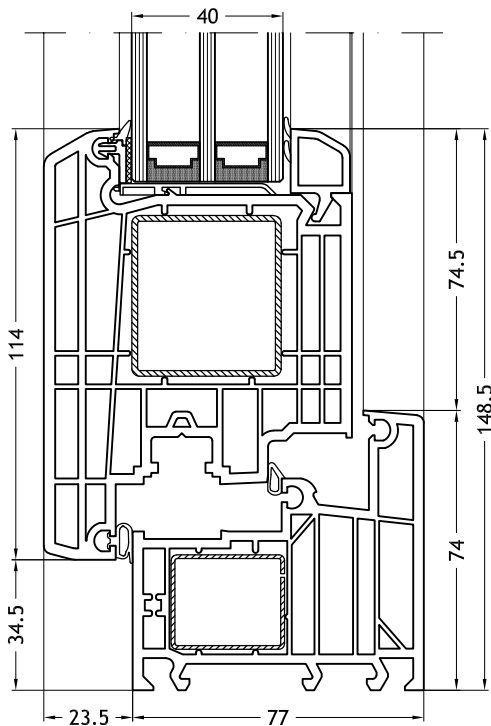
Marco L - 961 con hoja Step-line Door out
