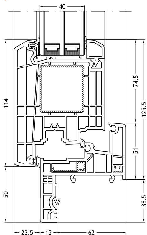
Marco Z, 965 con hoja Step-line Door out
