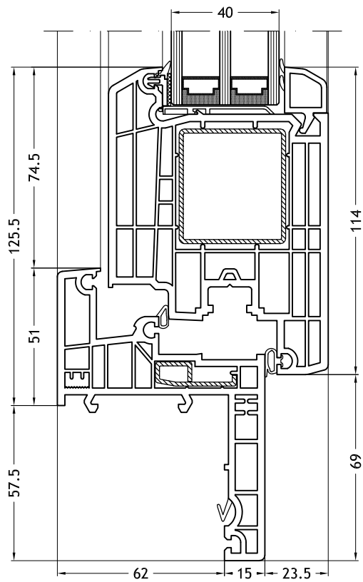
Marco Z, 966 con hoja Step-line Door
