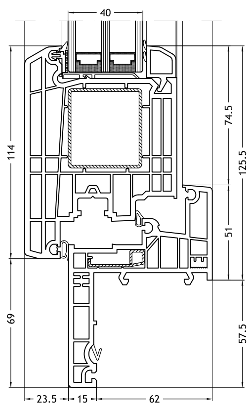
Marco Z, 966 con hoja Step-line Door out
