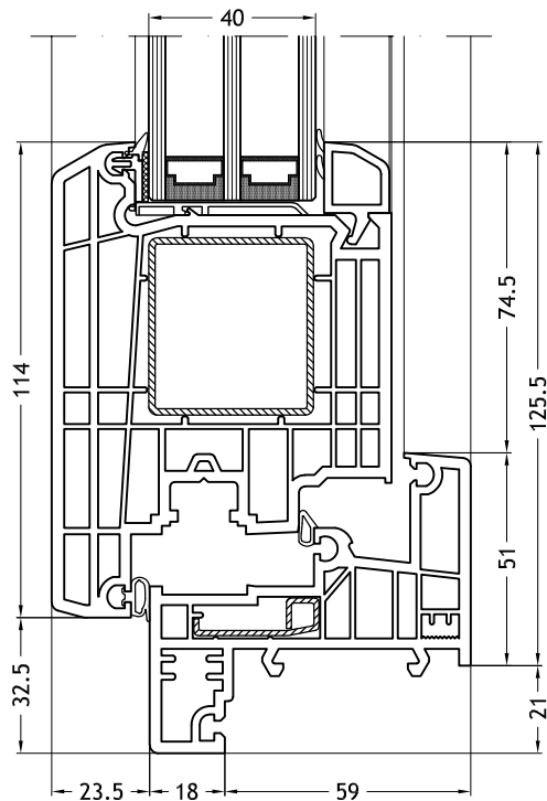
Marco Z, 964 con hoja Step-line Door out
