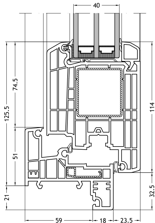
Marco Z, 964 con hoja Step-line Door
