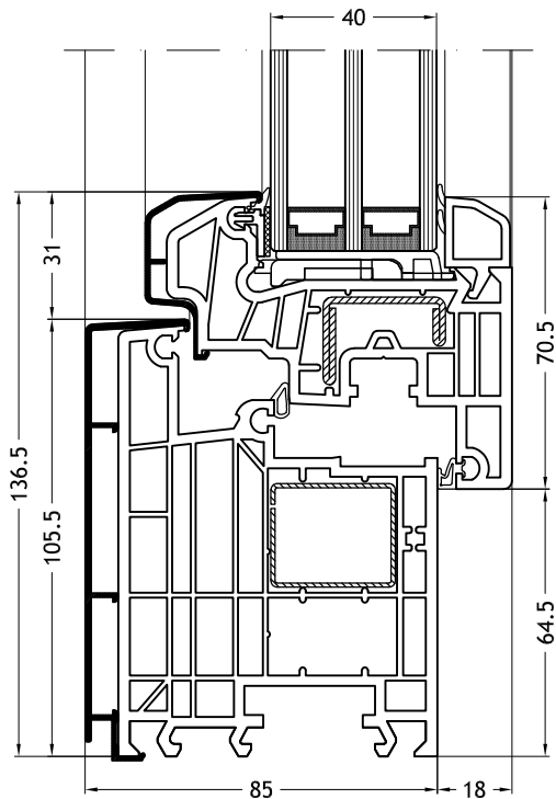
Blendrahmen L-Form 963N mit Flügel Classic-line
