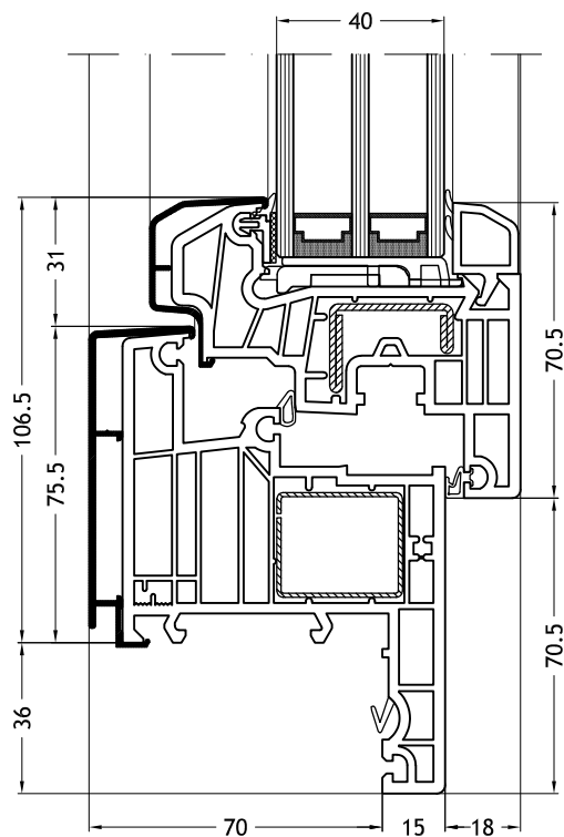
Blendrahmen Z-Form 967N mit Flügel Classic-line
