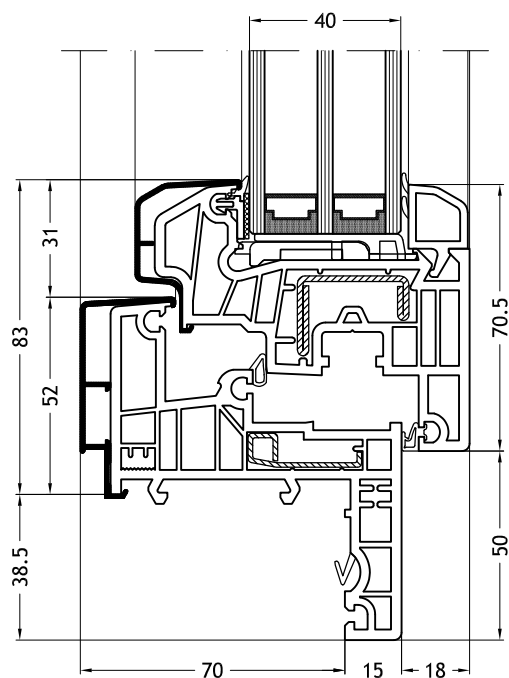
Blendrahmen Z-Form 965N mit Flügel Classic-line
