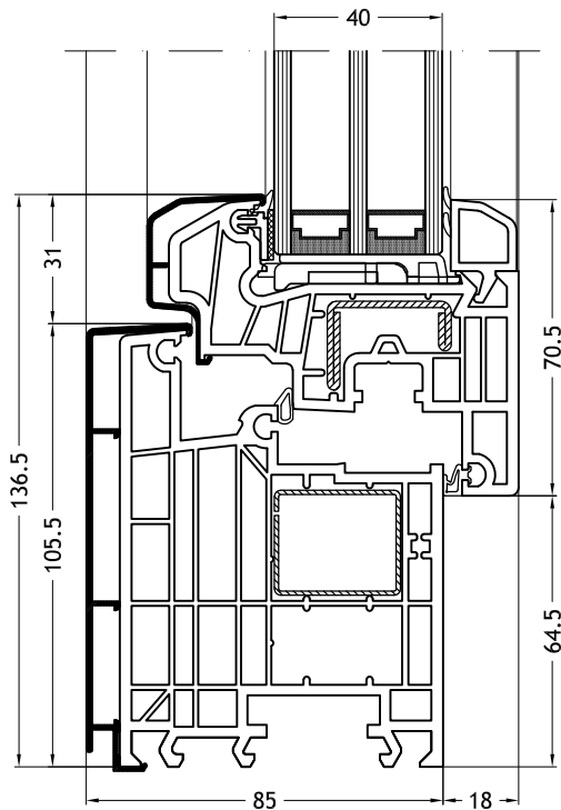
Telaio a L 963N con anta Classic-line
