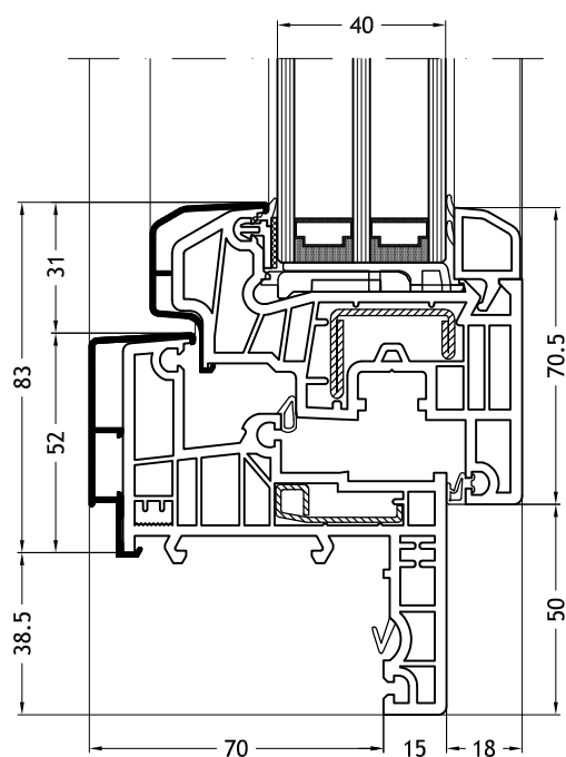
Telaio a Z 965N con anta Classic-line
