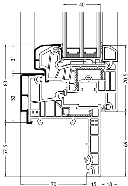
Telaio a Z 966N con anta Classic-line
