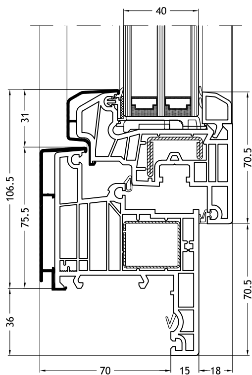
Telaio a Z 967N con anta Classic-line
