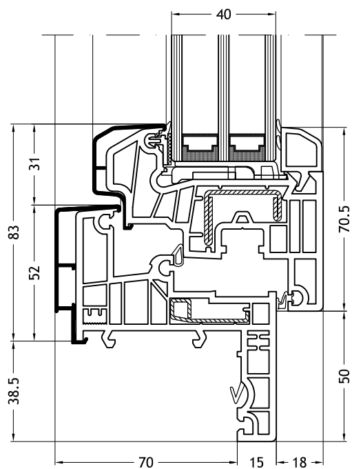
Kozijn Z-vorm 965N met vleugel Classic-line
