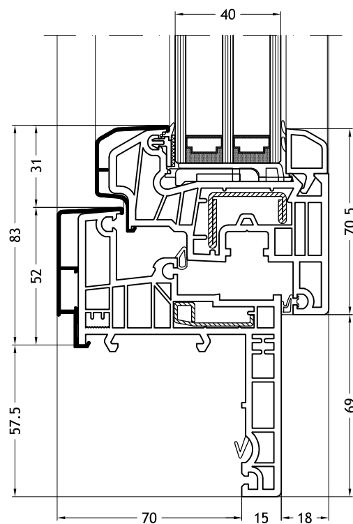
Kozijn Z-vorm 966N met vleugel Classic-line
