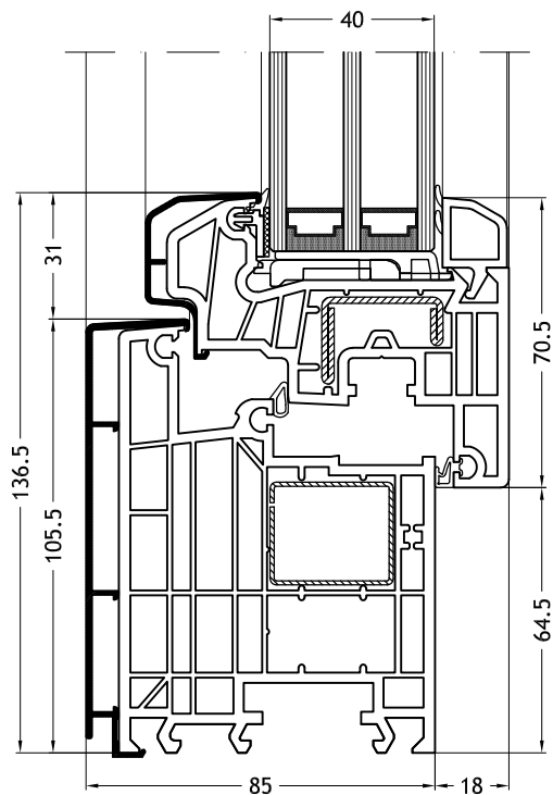
Kozijn L-vorm 963N met vleugel Classic-line
